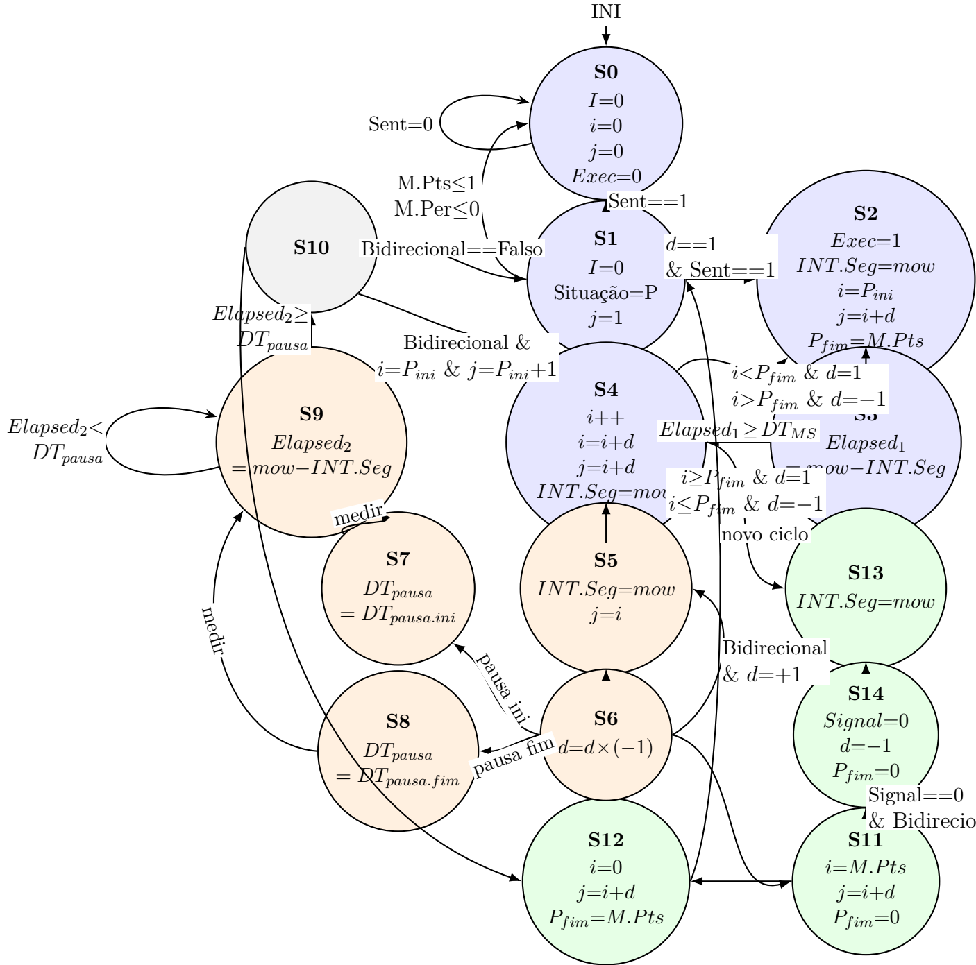
Figura 4.2: Esquema da FSM_Motion_Update .
