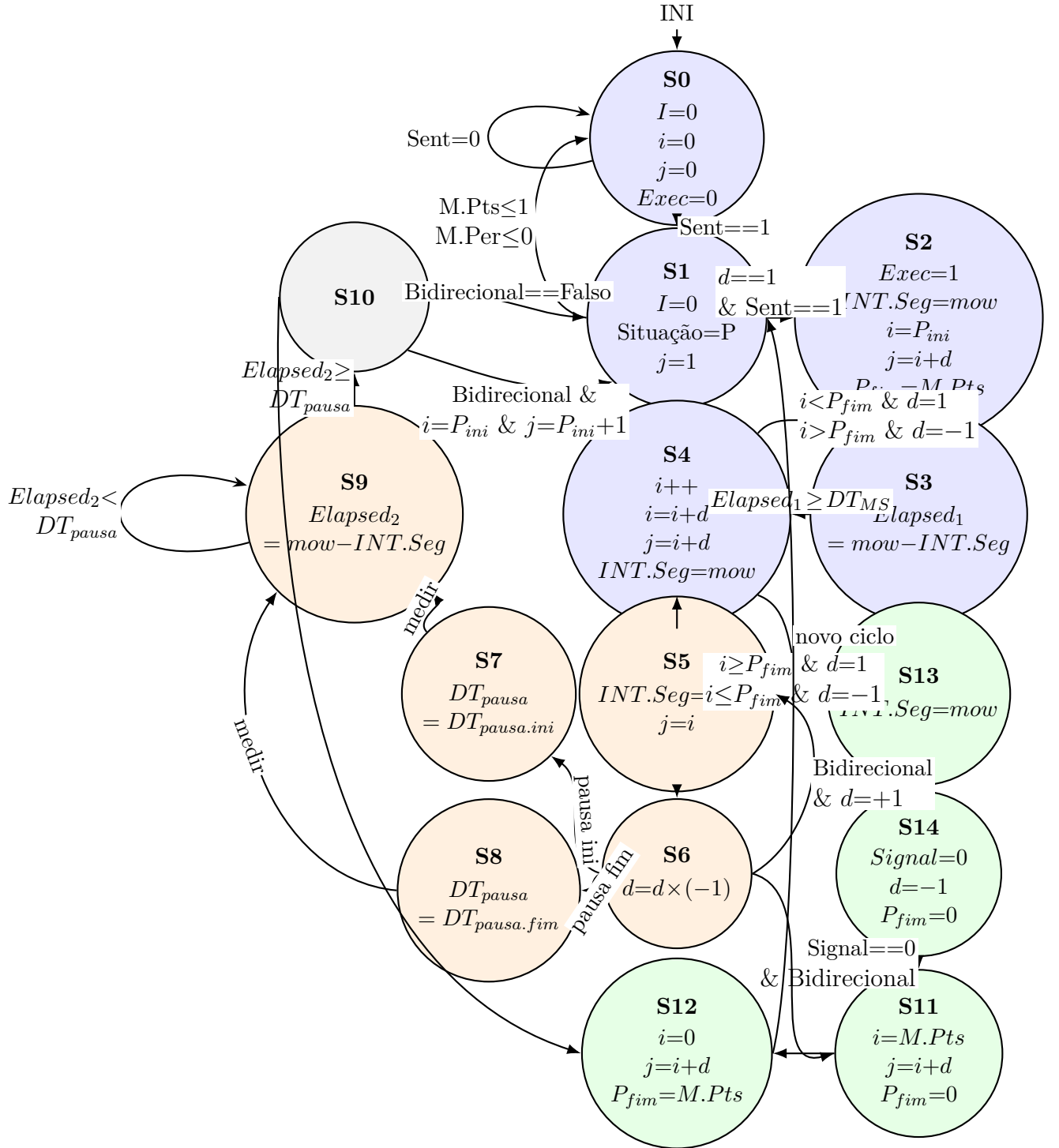
Figura 4.2: Esquema da FSM_Motion_Update .
