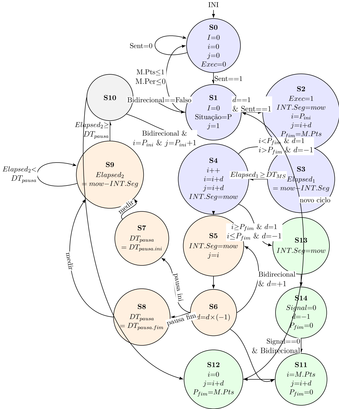
Figura 4.2: Esquema da FSM_Motion_Update .
