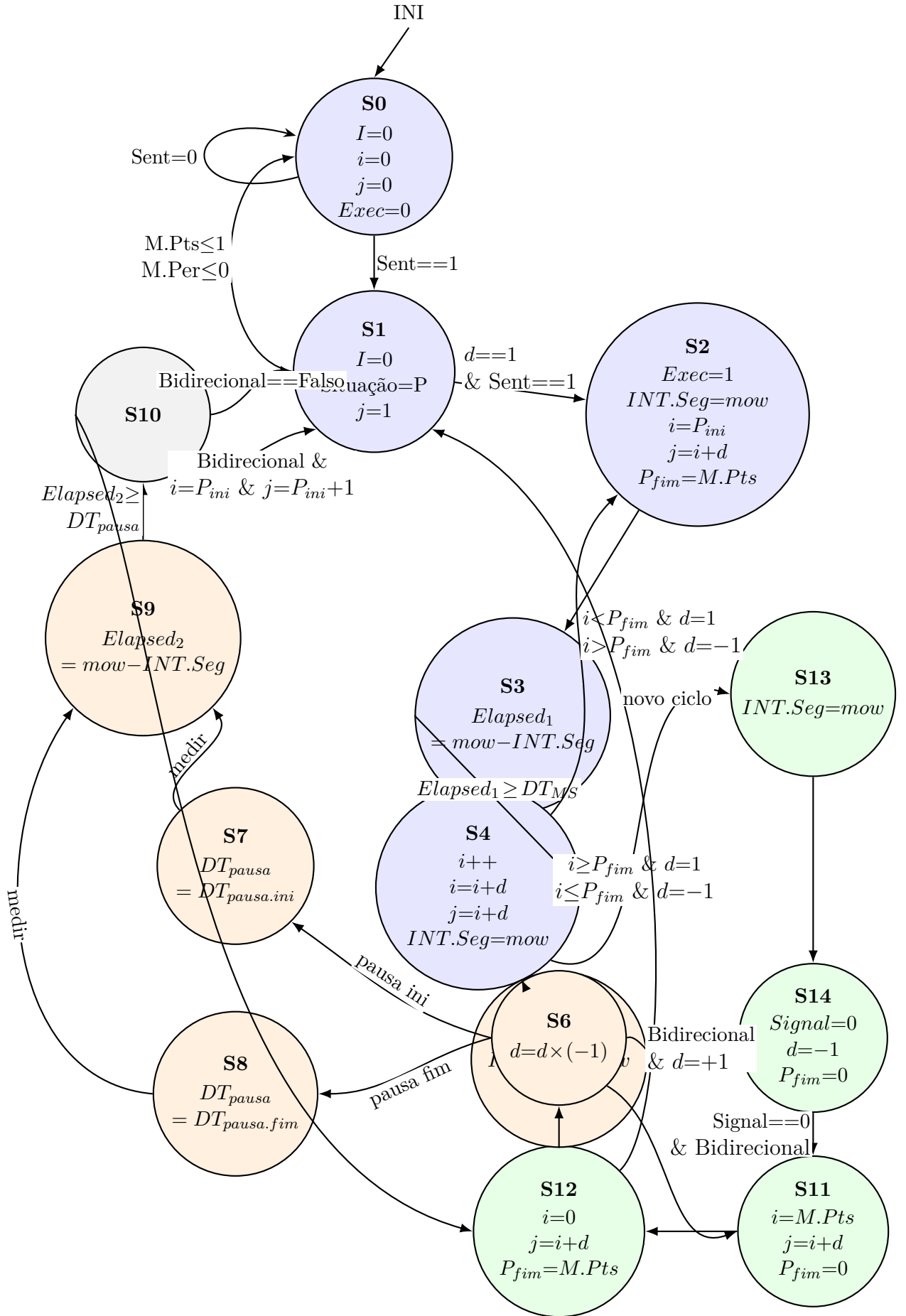
Figura 4.2: Esquema da FSM_Motion_Update .
