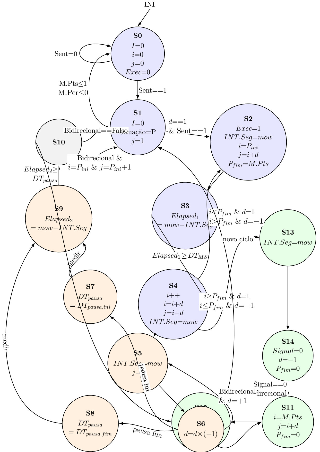
Figura 4.2: Esquema da FSM_Motion_Update .
