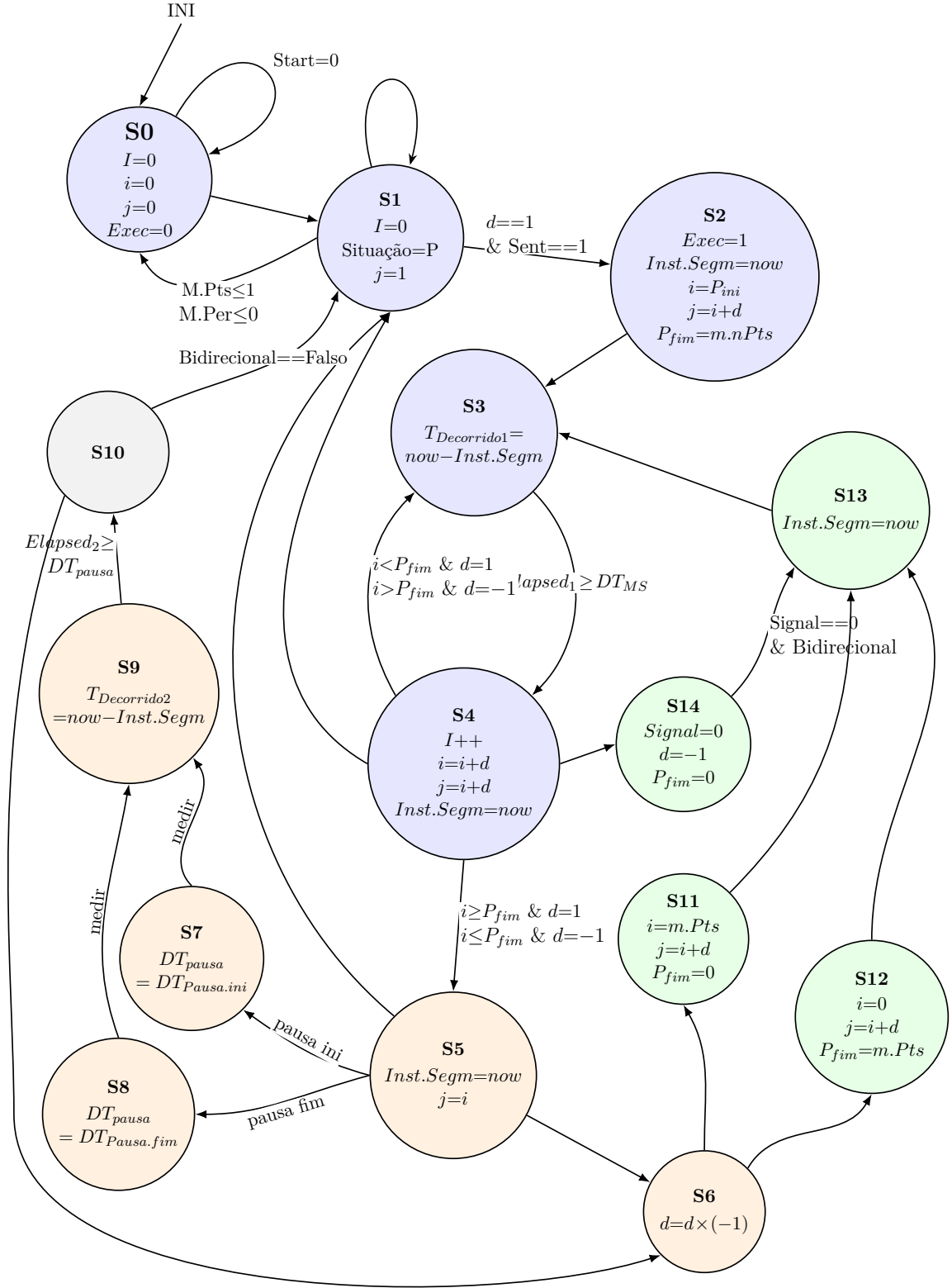
Figura 4.2: Esquema da FSM_Motion_Update.
