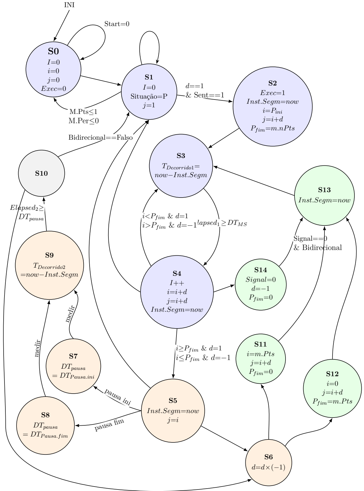
Figura 4.2: Esquema da FSM_Motion_Update .
