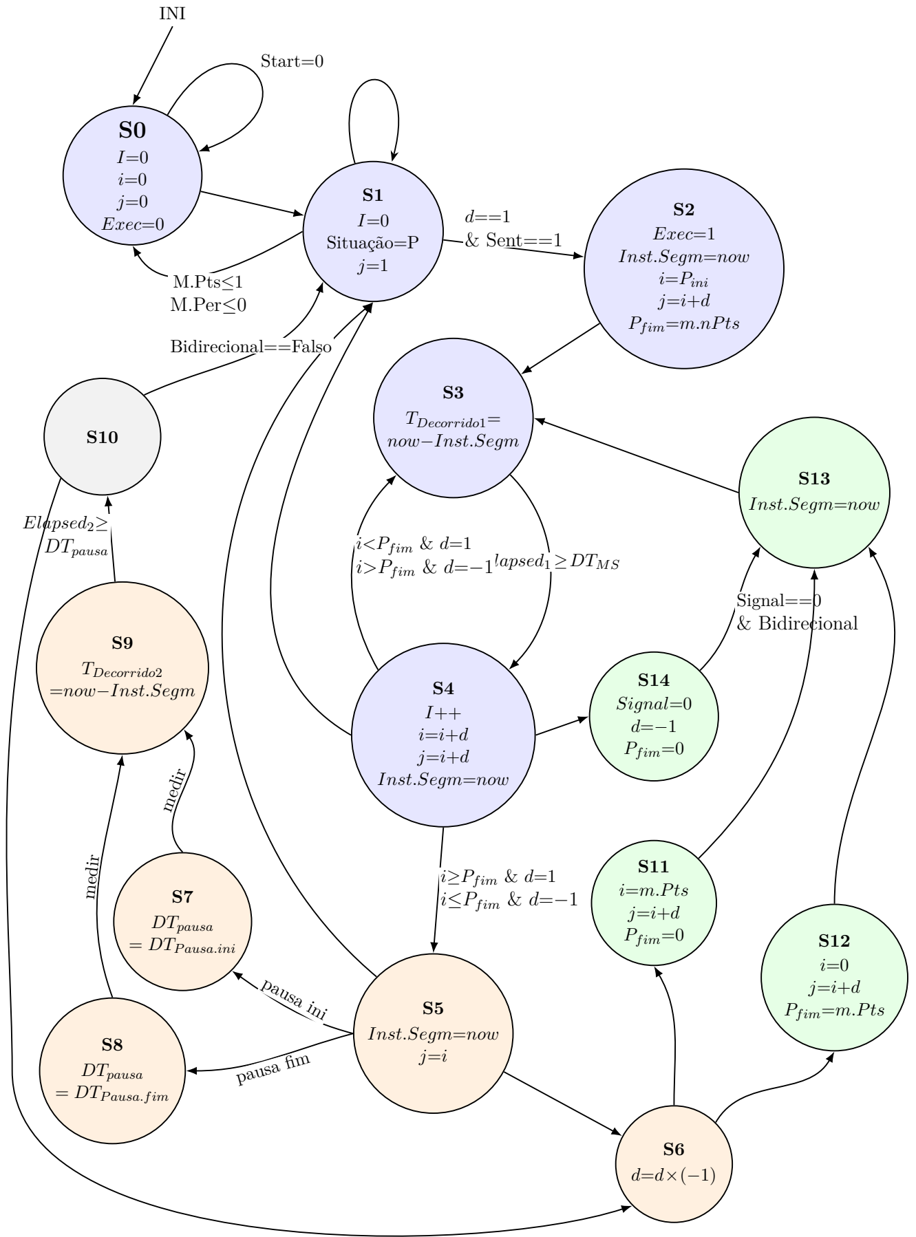
Figura 4.2: Esquema da FSM_Motion_Update.
