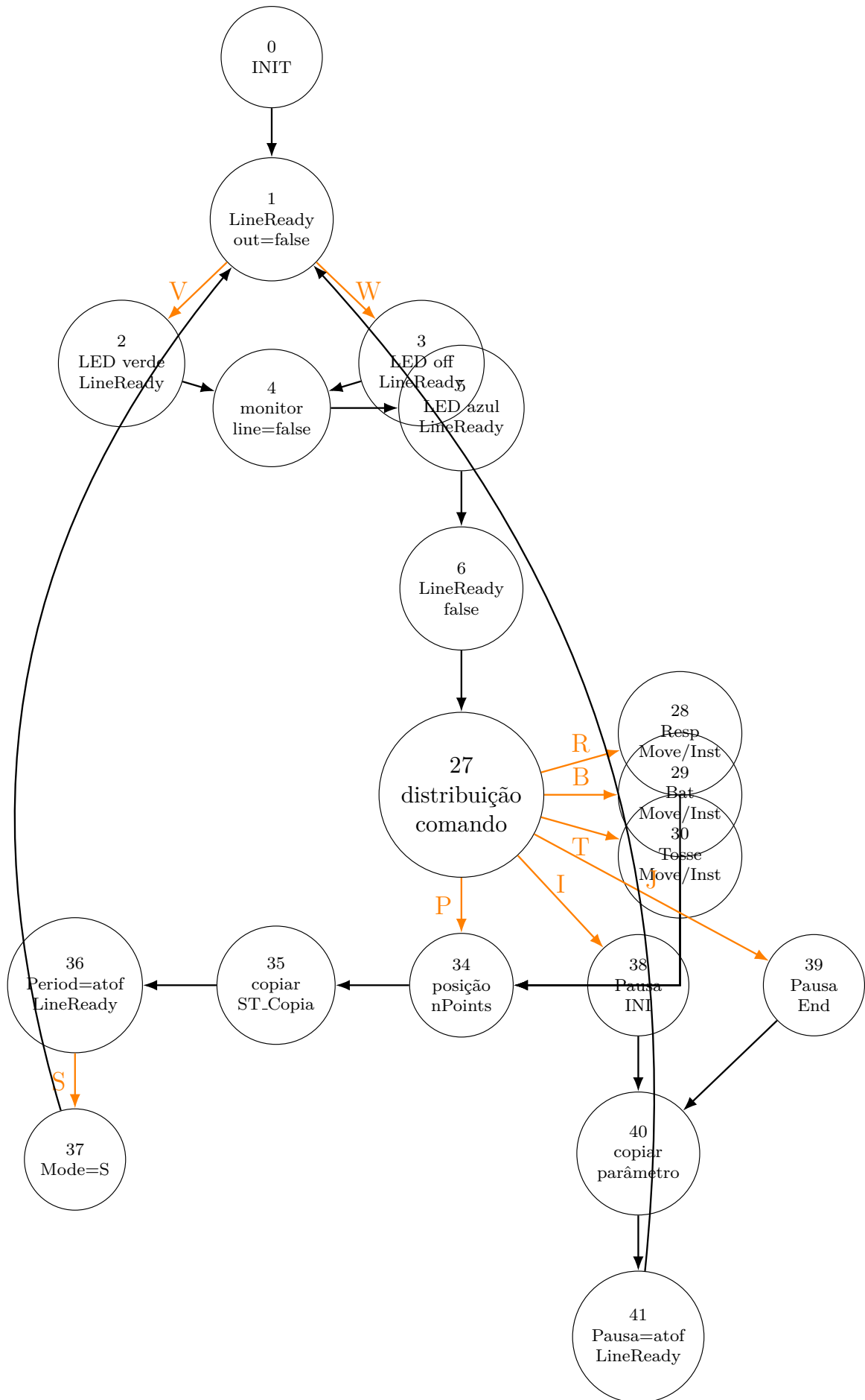
Figura 4.6: FSM.Serial_Command redesenhada a partir dos esquemas das páginas 46 e 47 das notas de projeto.
