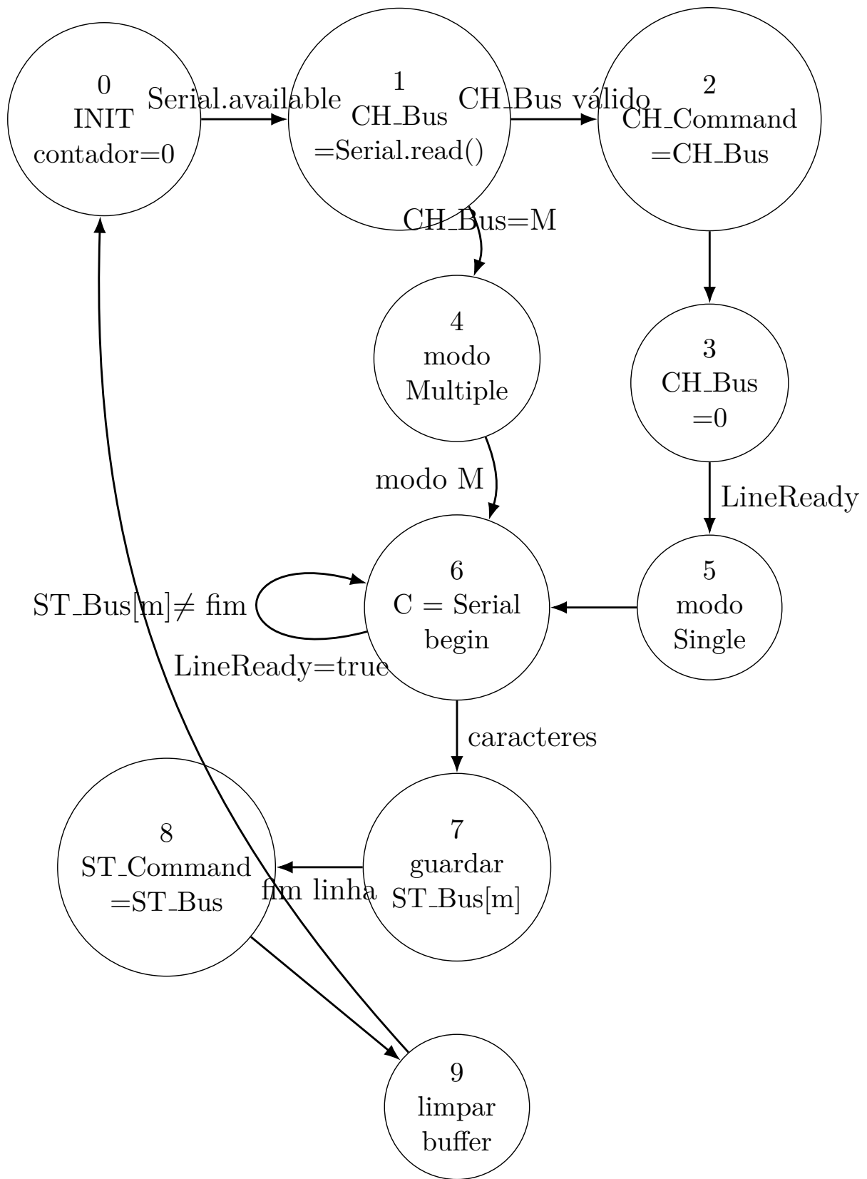
Figura 4.5: FSM_Serial_Read redesenhada a partir do esquema da página 44 das notas de projeto.
