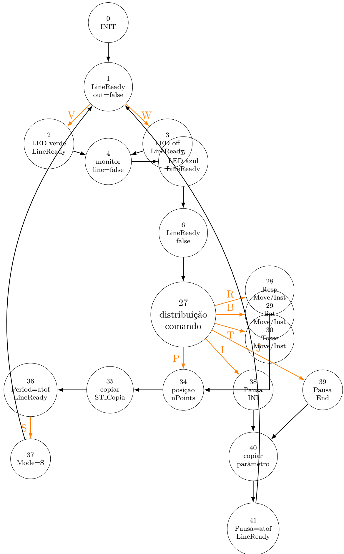
Figura 4.7: FSM_Serial_Command redenhada a partir dos esquemas das páginas 46 e 47 das notas de projeto.
