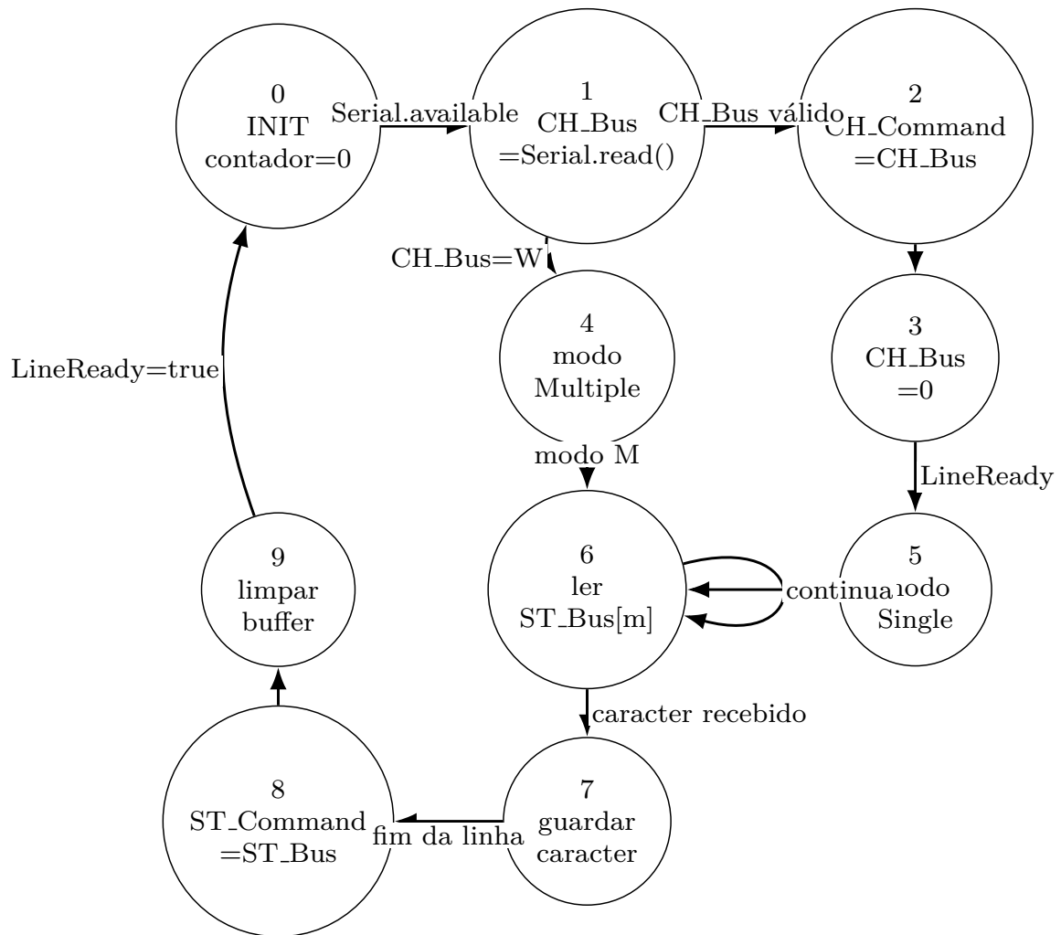
Figura 4.6: FSM_Serial_Read redesenhada a partir do esquema da página 44 das notas de projeto.
