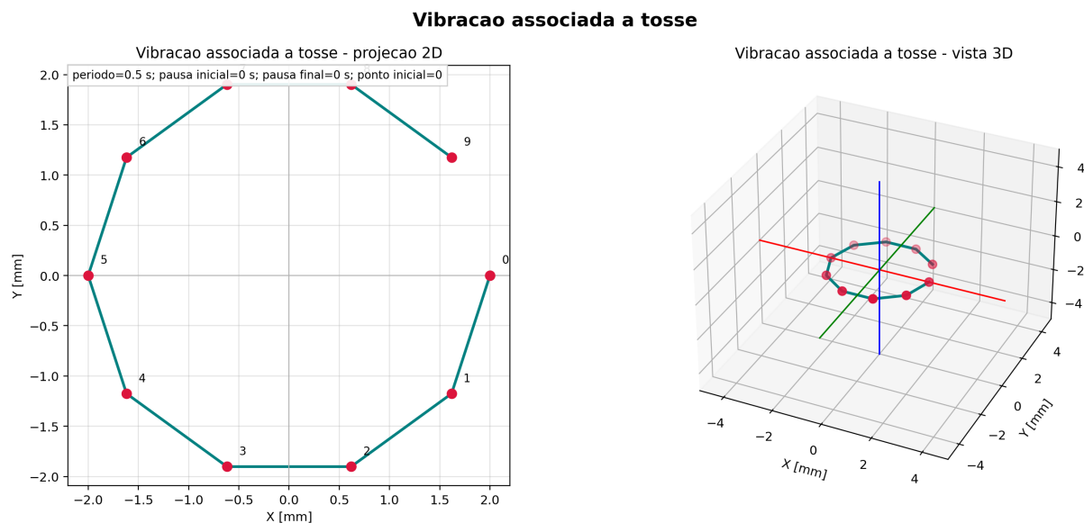
Figura 4.5: Trajetória calculada para a vibração associada à tosse, com representação 2D e 3D dos pontos de passagem.
