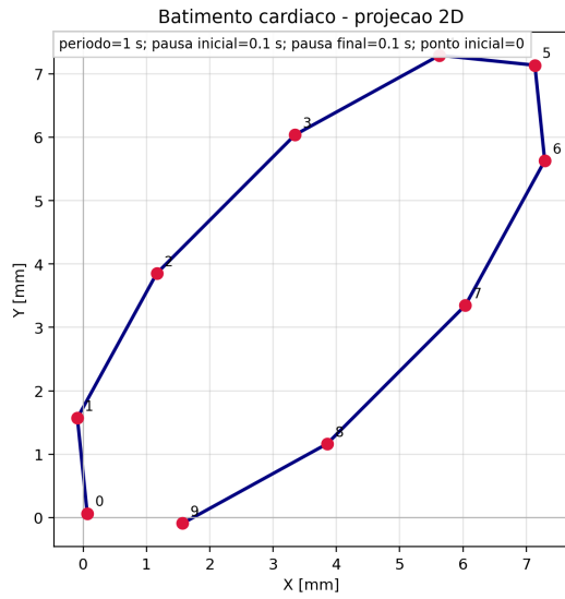
Figura 4.3: Trajetória calculada para o movimento de batimento cardíaco, com representação 2D e 3D dos pontos de passagem.
