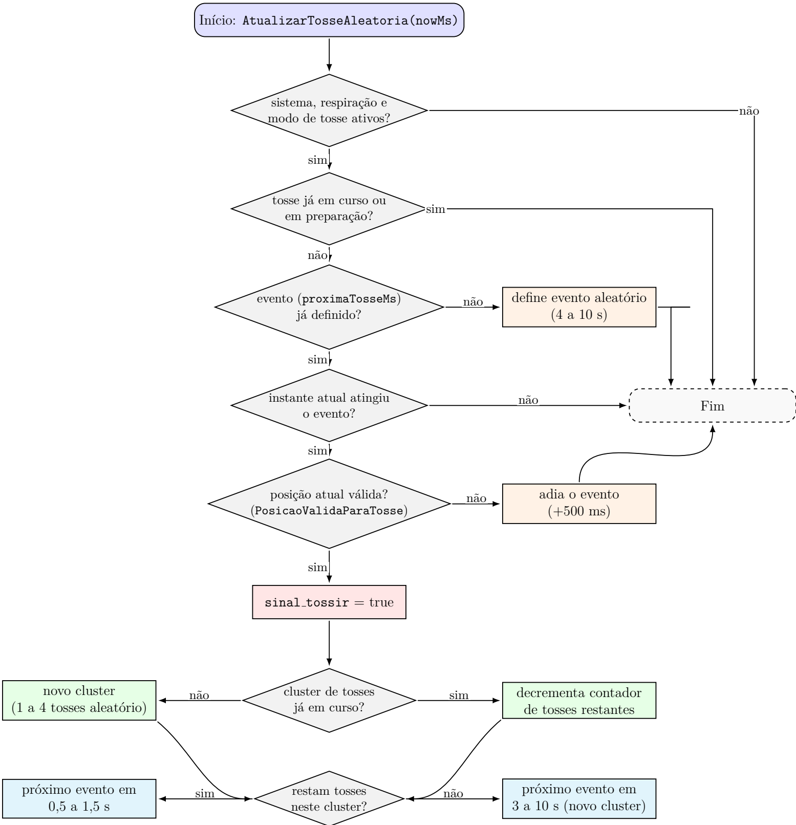
Figure 1: Fluxograma da função AtualizarTosseAleatoria().
