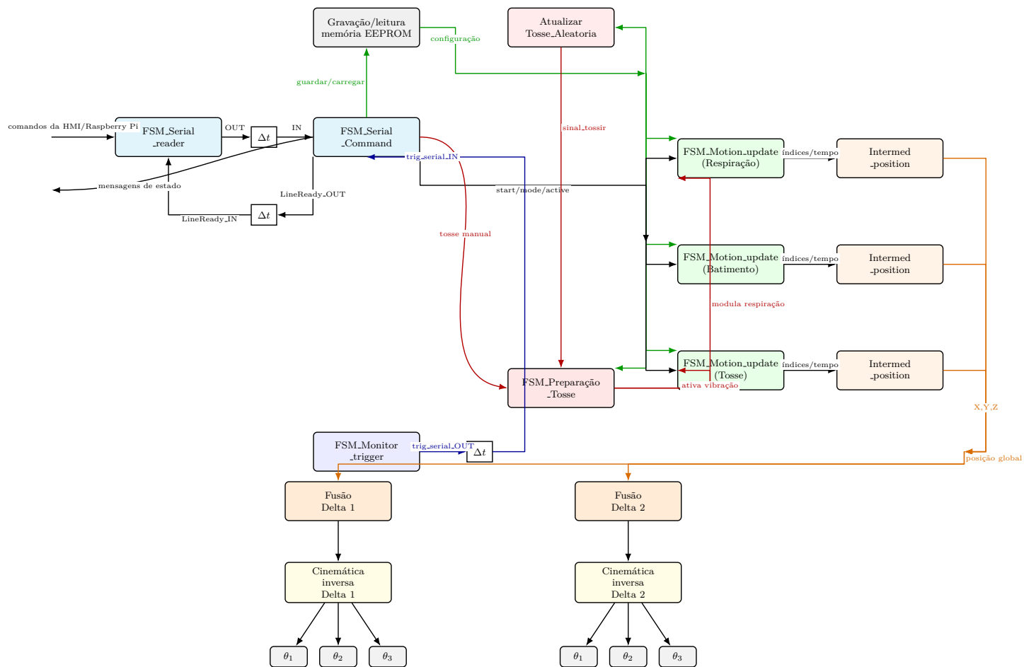
Figure 1: Estrutura global das máquinas de estados e blocos de controlo do firmware, com os atrasos de um ciclo representados por \Delta t .
