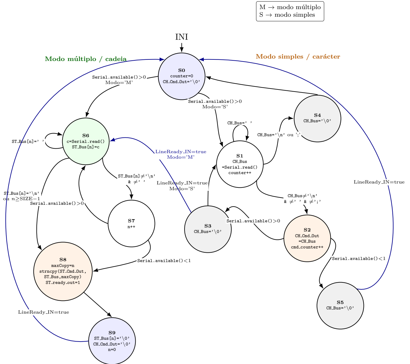
Figure 1: Esquema da FSM_Serial_Reader.
