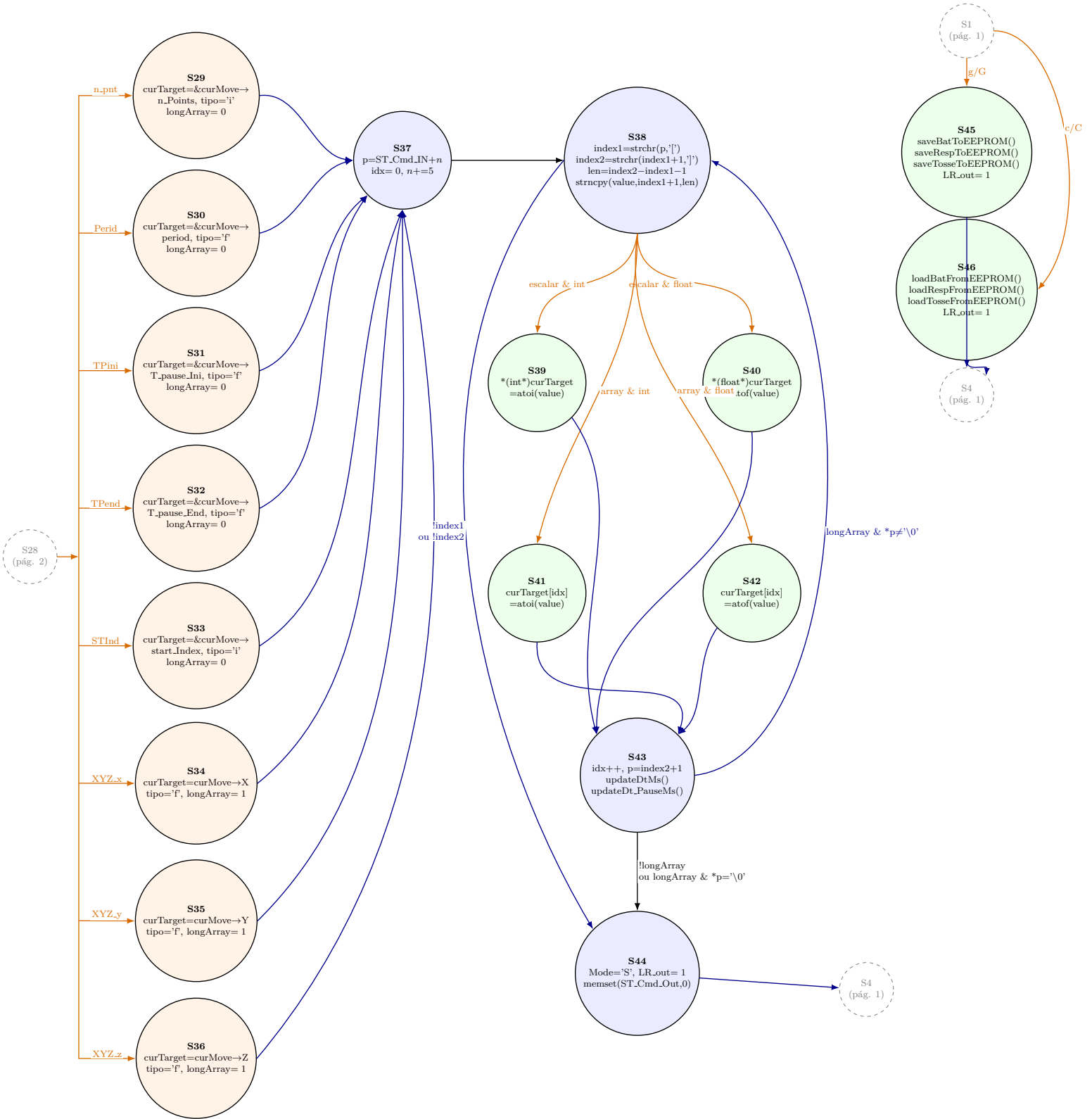
Figure 1: FSM_Serial_Command (parte 3 de 3): seleção de campo, escrita do valor e comandos de EEPROM.
