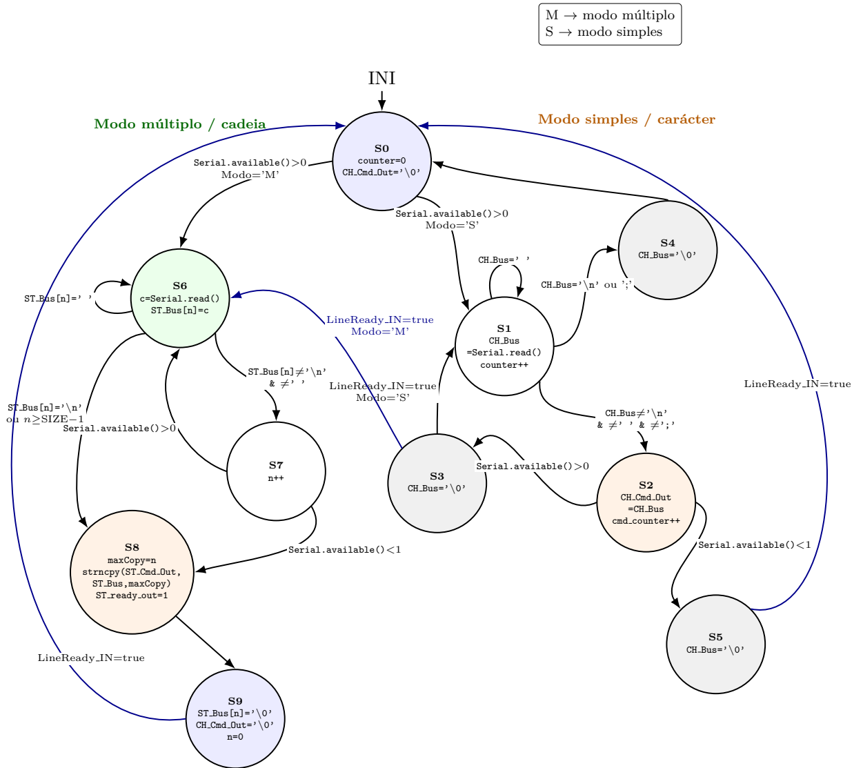
Figure 1: Esquema da FSM_Serial_Reader.
