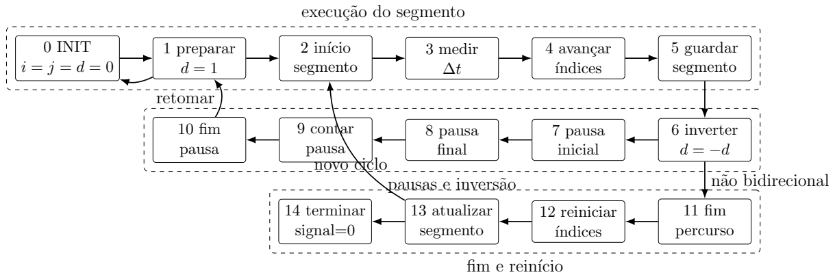
Figura 4.2: FSM_Movement redesenhada a partir do esquema da página 38 das notas de projeto.
