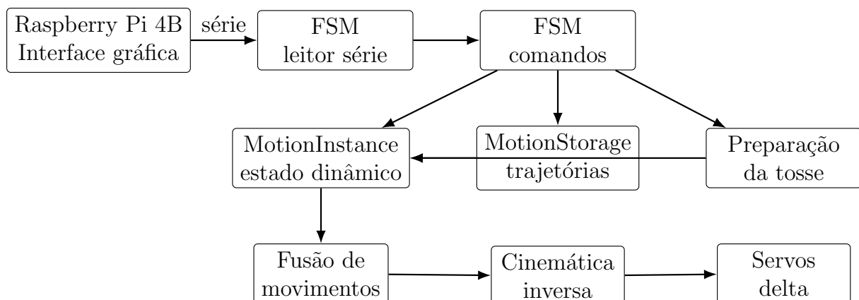
Figura 4.1: Arquitetura geral de software e fluxo de controlo do protótipo.
