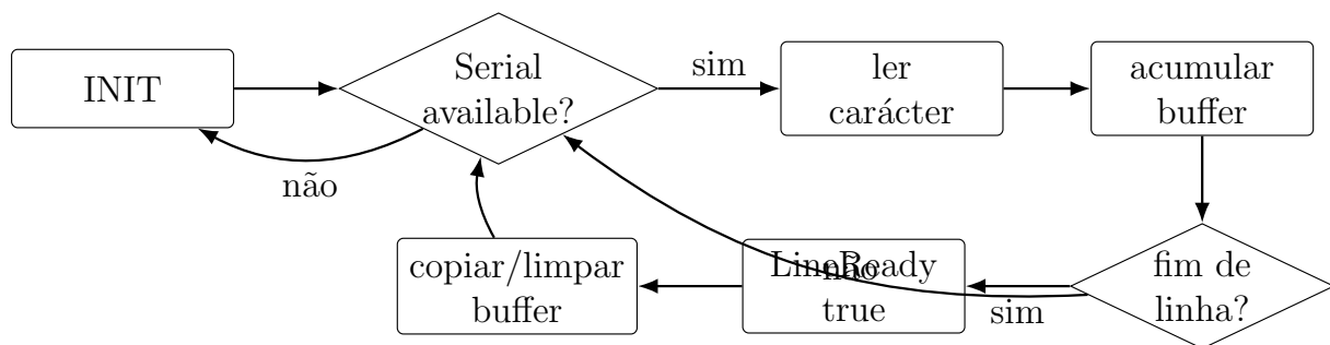
Figura 4.3: Representação simplificada da máquina de estados do leitor série.
