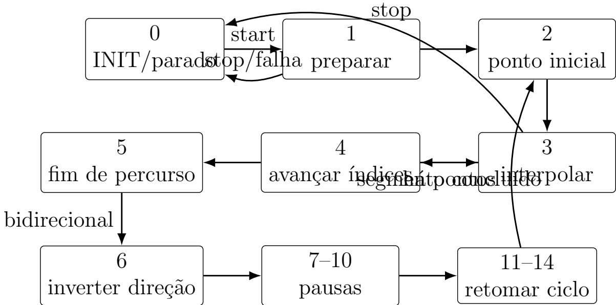
Figura 4.2: Representação simplificada da máquina de estados de movimento.
