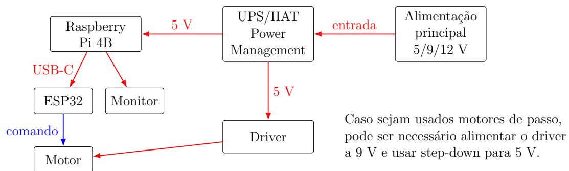
Figura 3.2: Esquema de alimentação com UPS/HAT e alternativa de alimentação para driver, baseado no esquema da página 30 das notas de projeto.
