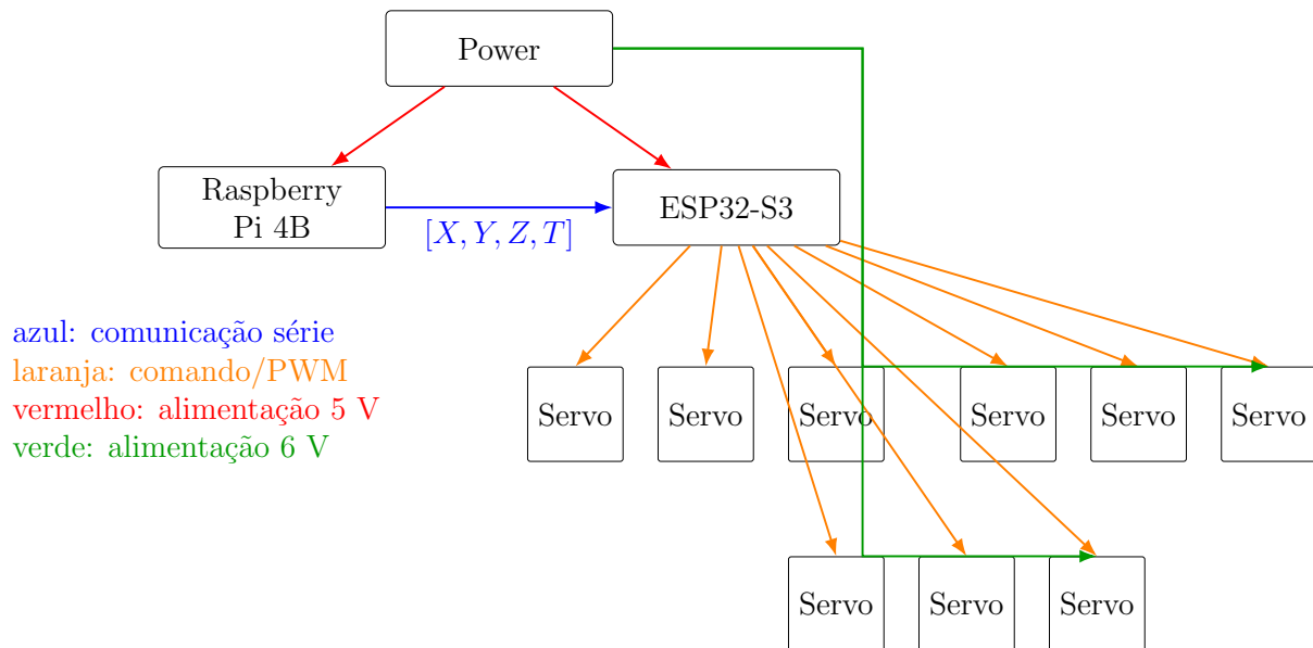
Figura 3.1: Esquema geral de alimentação e comunicação entre Raspberry Pi, ESP32-S3 e servos, baseado no esquema da página 27 das notas de projeto.
