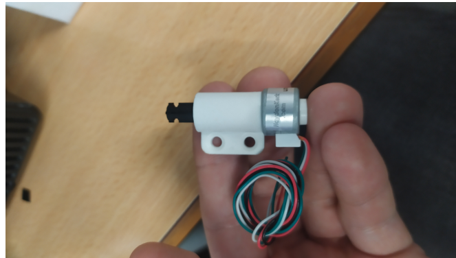
Figura 3.3: Servo motor com suporte impresso em 3D para validação do acoplamento mecânico com a estrutura do manipulador delta, março de 2026.
