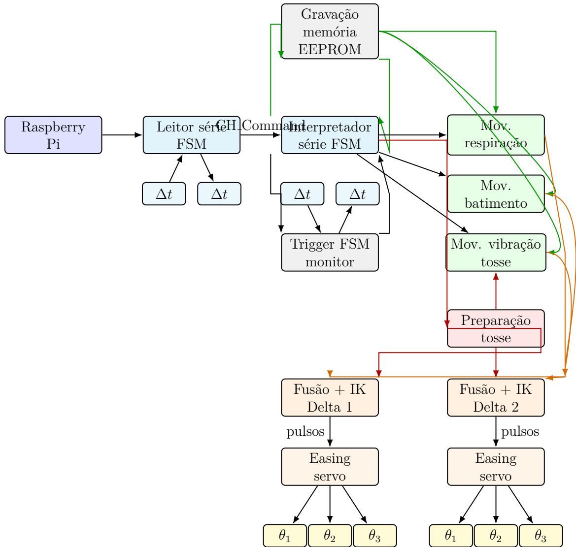
Figura 4.1: Estrutura global das máquinas de estados e blocos de controle.
