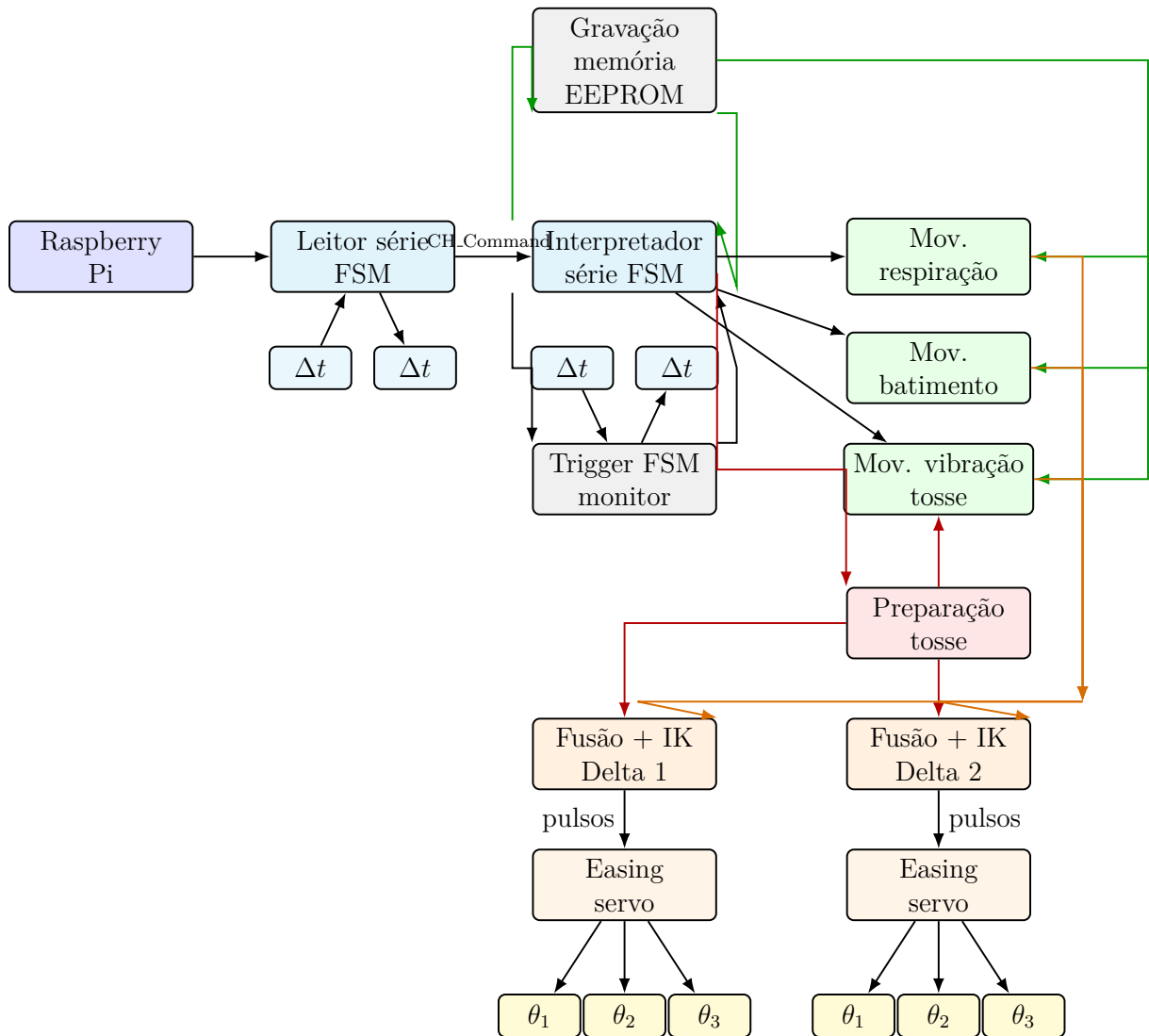
Figura 4.1: Estrutura global das máquinas de estados e blocos de controle.
