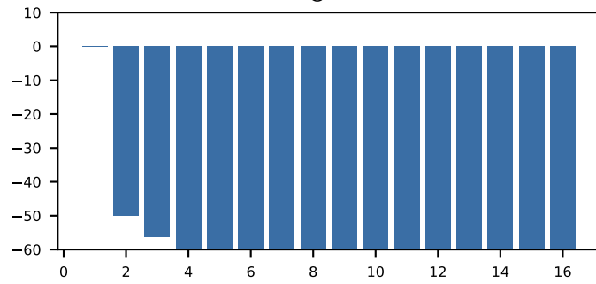
G3 @ 154.74s
