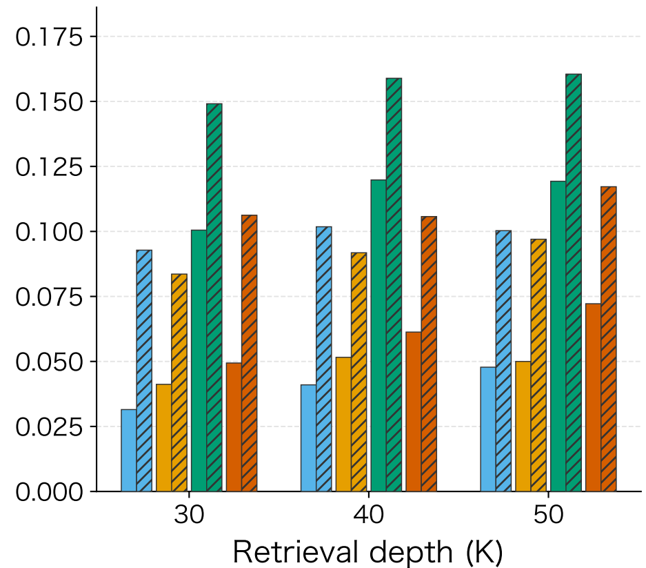
FeTaQA
