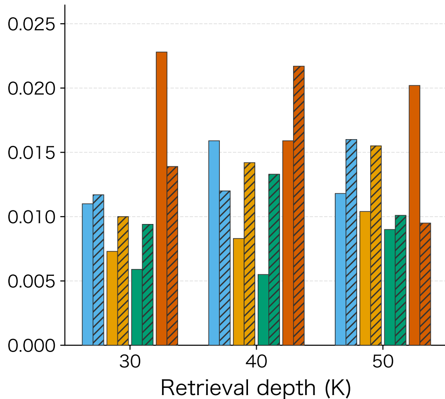
OTTQA
