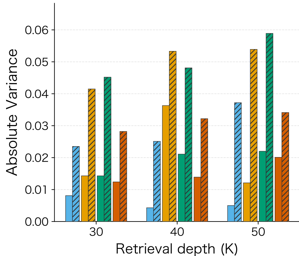
E2E-WTQ
