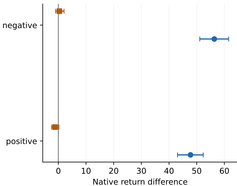
Pendulum
