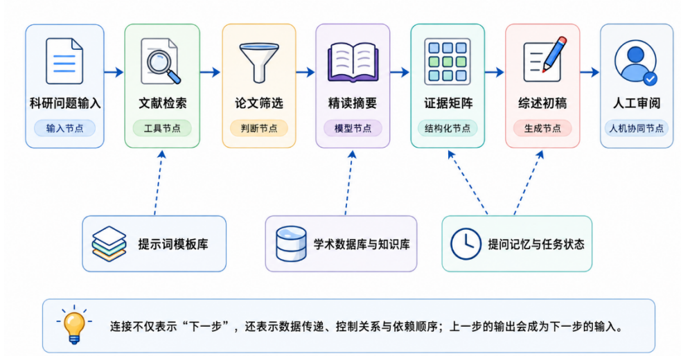
图 7-11 智能体 workflows 中的节点与连接逻辑
