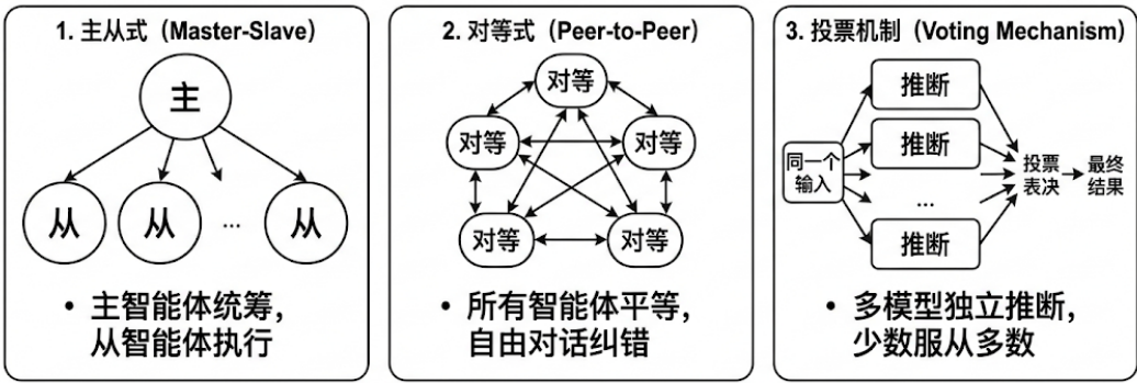
图 7-12 多智能体协作模式
