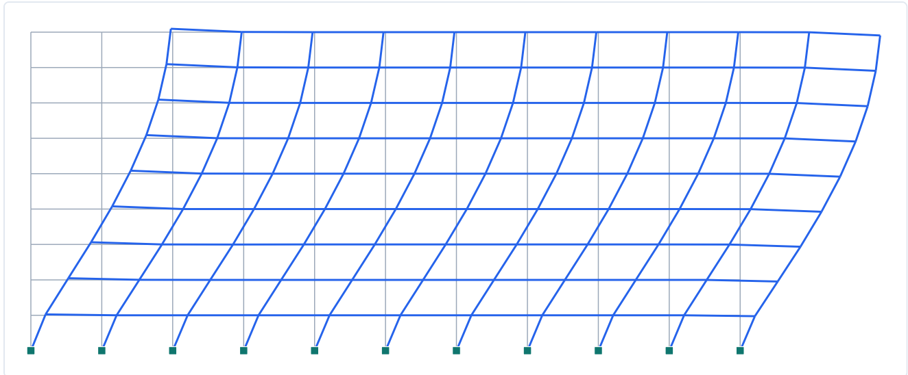
*Figura 1. Modo 1 ( \omega^2 = 0.5899 , T = 8.18 s) — primer modo de oscilación lateral del pórtico.*
