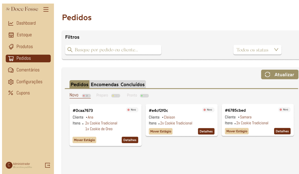
Figura 17 – Protótipo no Figma - Tabela de pedidos (Admin)
