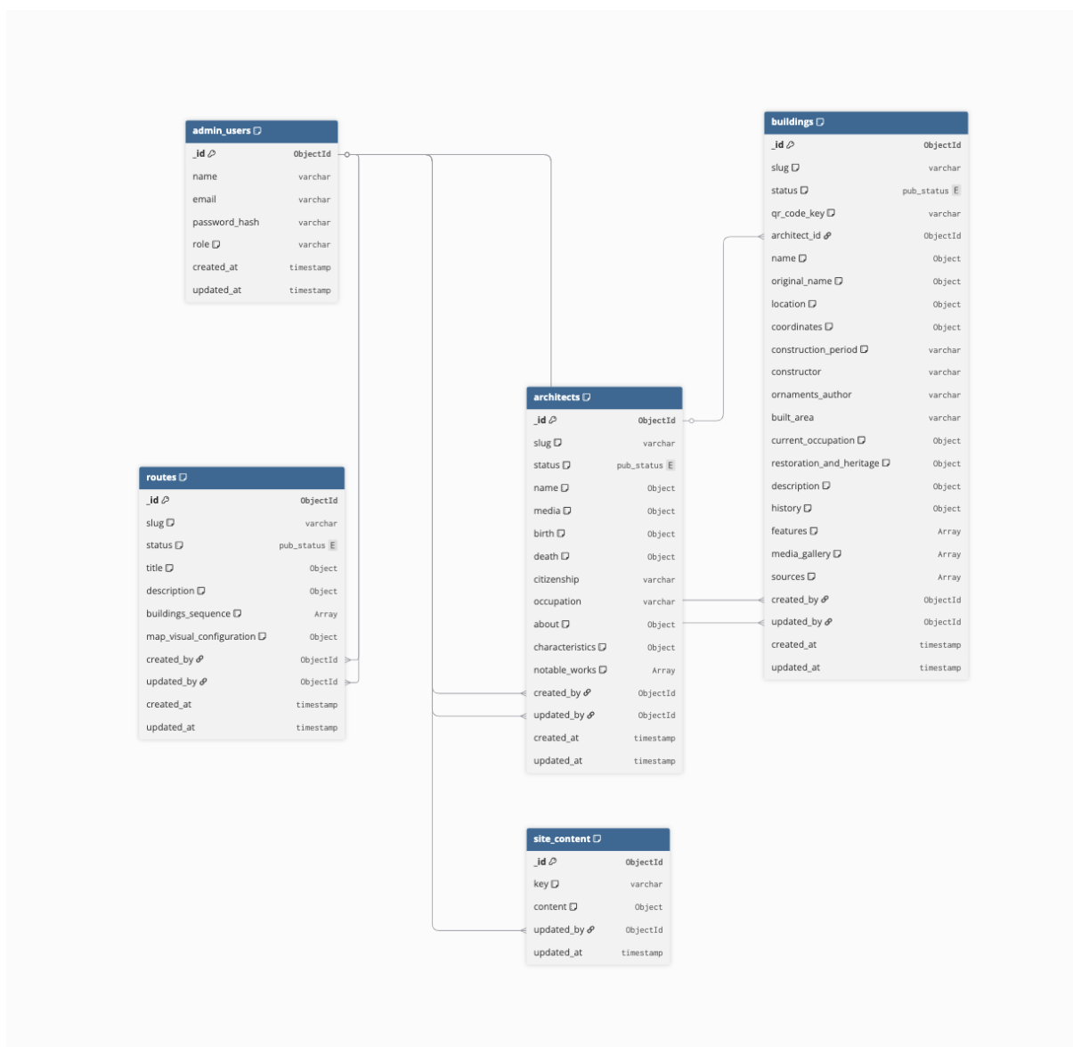
Figura 20 – Diagrama do Banco de Dados
