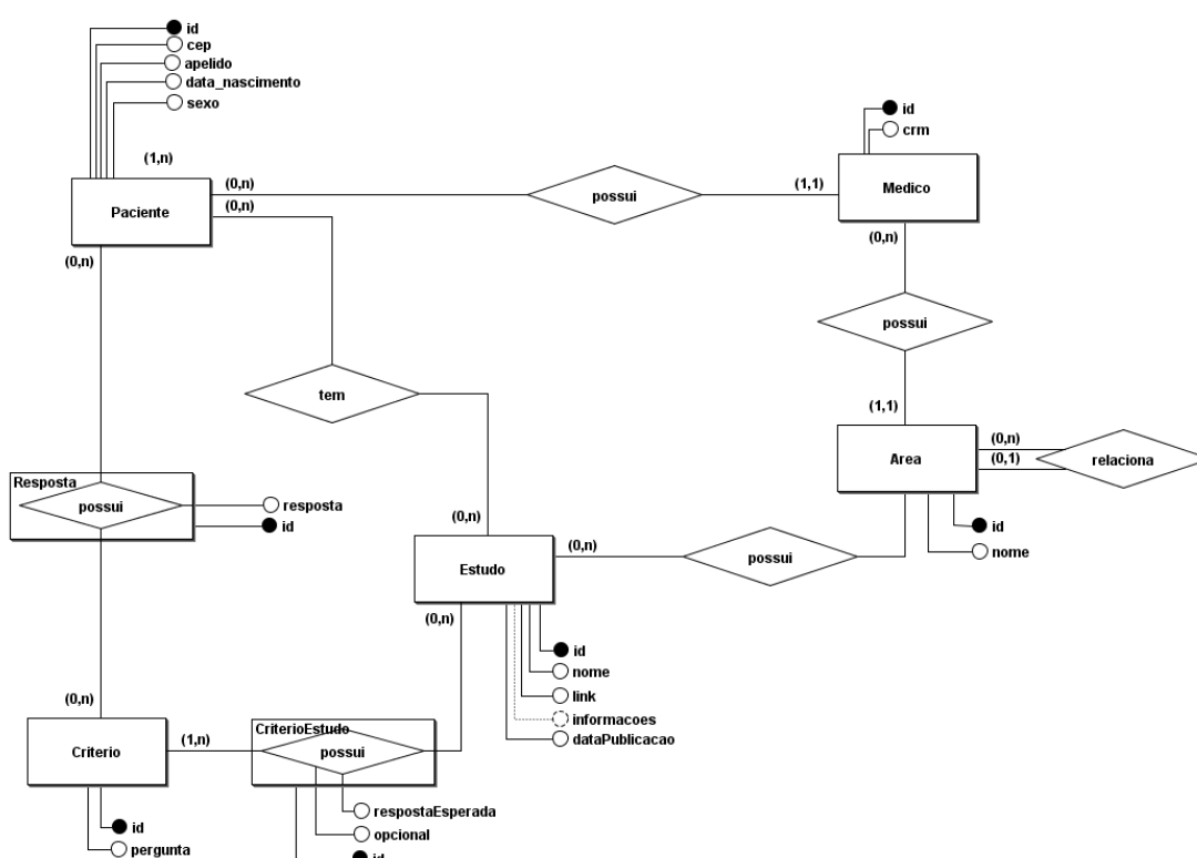
Figura 7 – Modelagem do banco de dados
