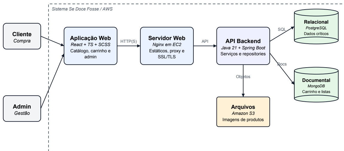
Figura 14 – Diagrama C4 de contêineres do projeto - AGES III
