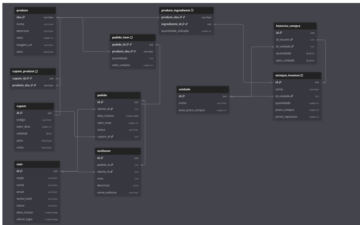
Figura 13 – Banco de Dados
