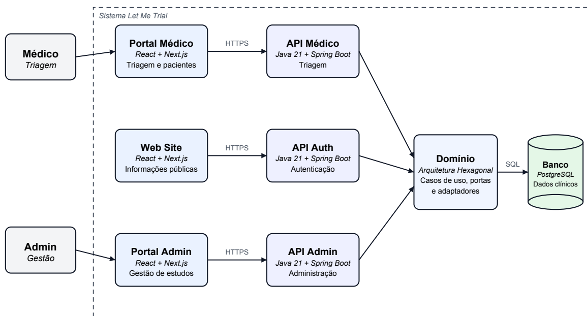
Figura 8 – Diagrama C4 de contêineres do projeto - AGES II
