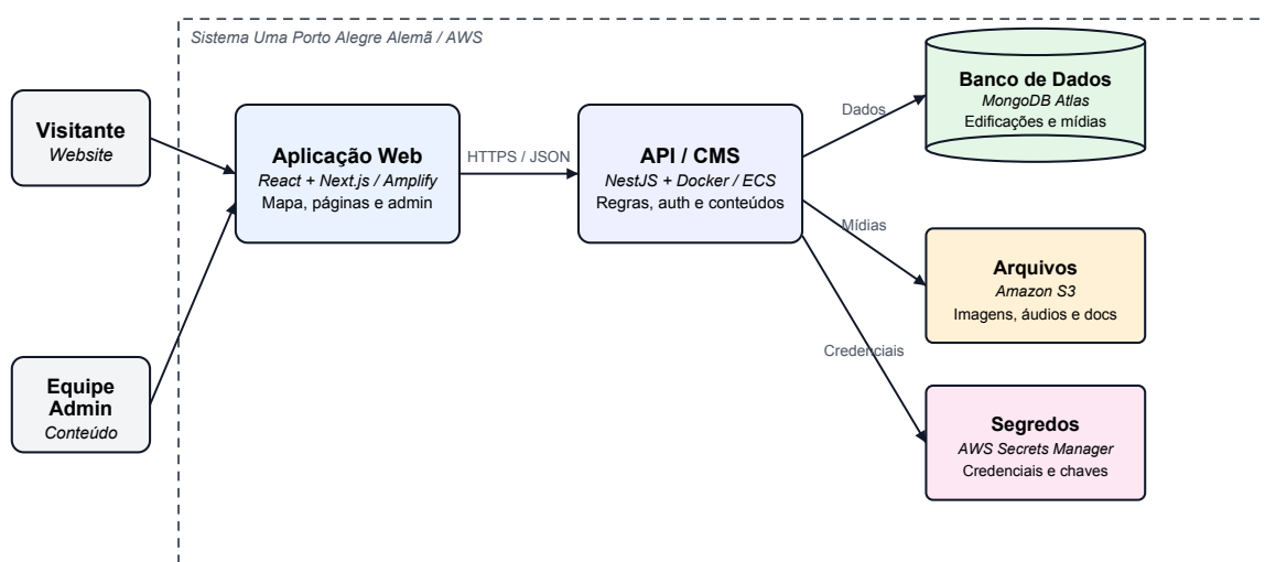
Figura 21 – Diagrama C4 de contêineres do projeto - AGES IV
