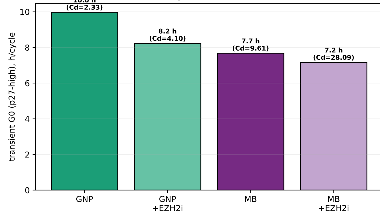
(d) EZH2 inhibition de-represses CyclinD1 and collapses the transient G0
