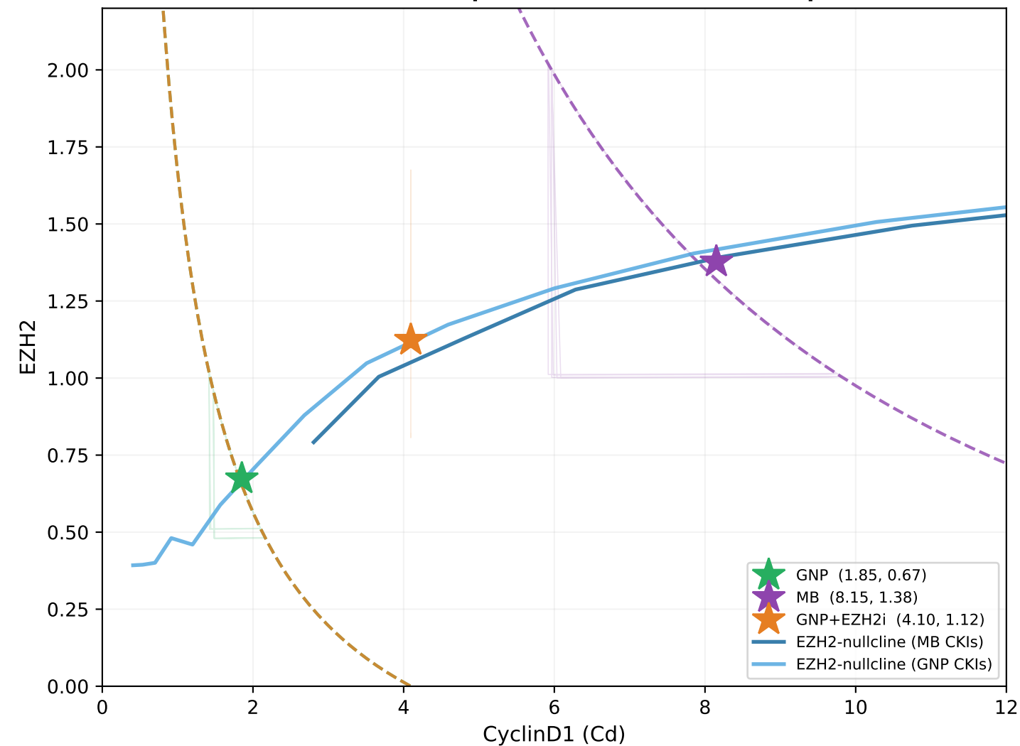
(D) Mitogen bifurcation: EZH2 feedback raises the mitogen threshold for proliferation (gated quiescence)
