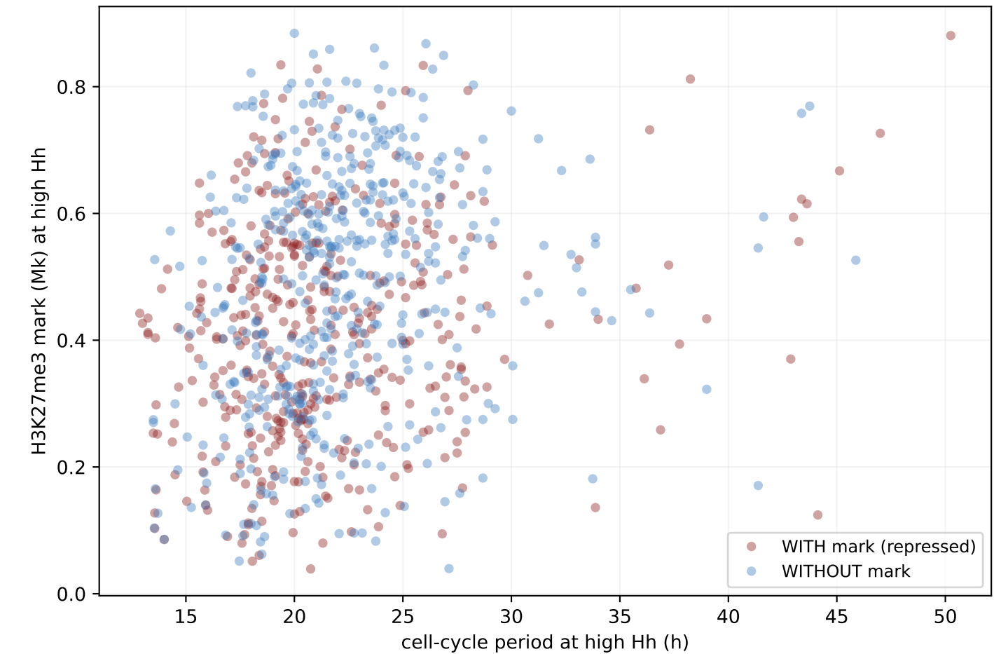
(D) The dilution-vs-restoration RACE (mu-distributed cells)
