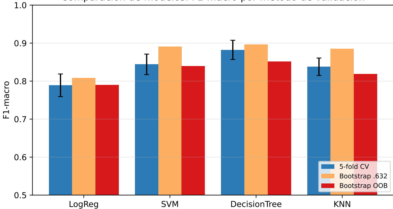
Comparación de modelos: F1-macro por método de validación
