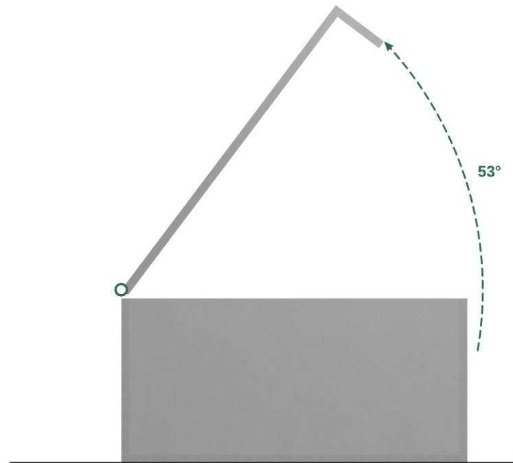
LEFT END Lid 53° · 1:3
