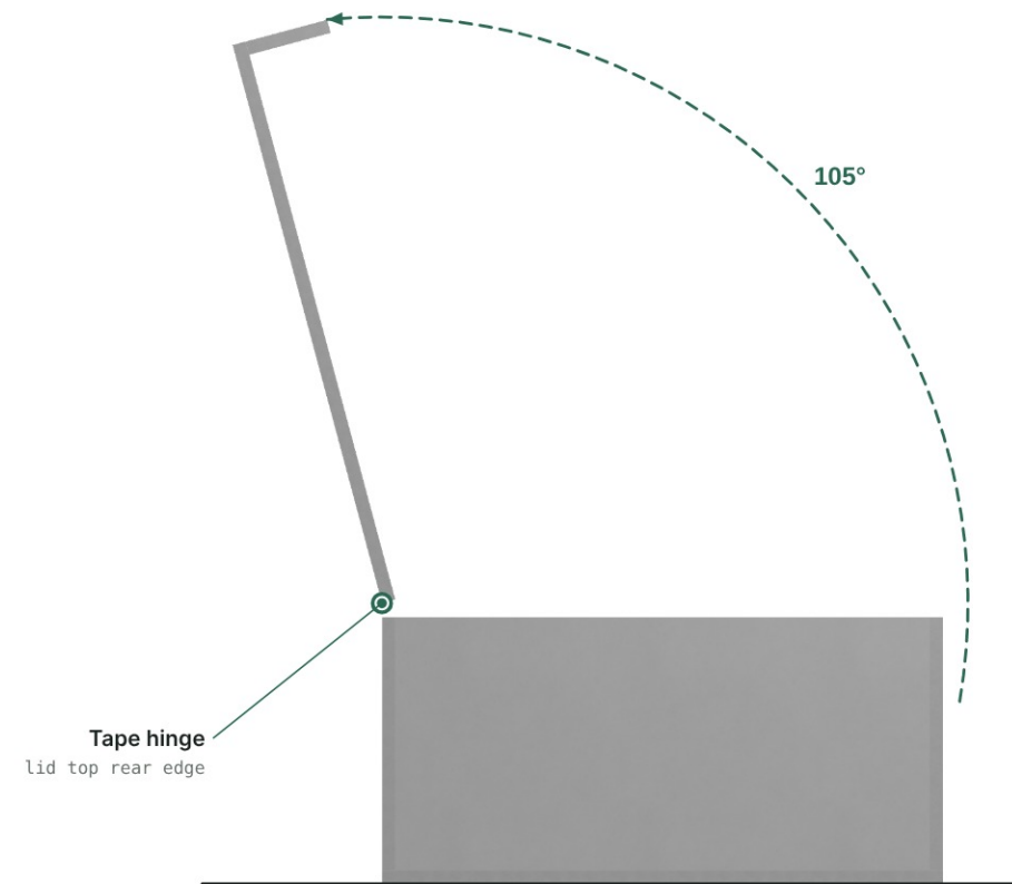
LEFT END Lid open 105° · 1:3
