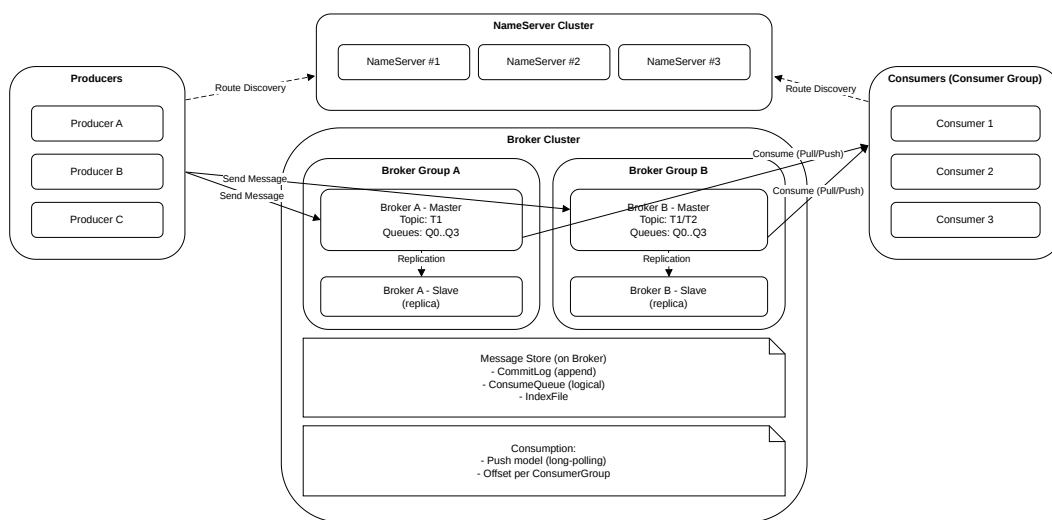
图 2-1: RocketMQ 架构图
