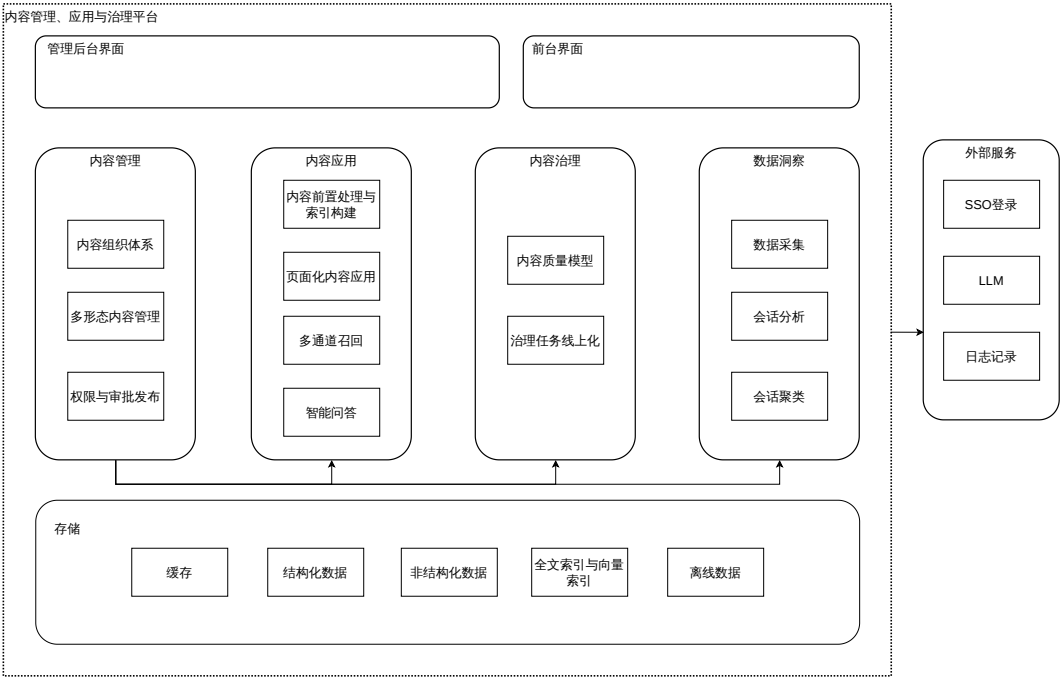
图 3-6: 逻辑视图
