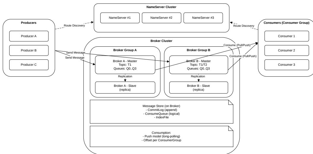
图 2-1: RocketMQ 架构图
