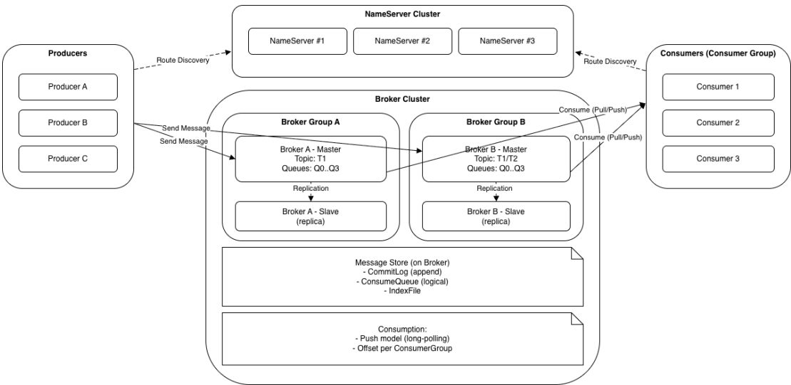
图 2-1: RocketMQ 架构图
