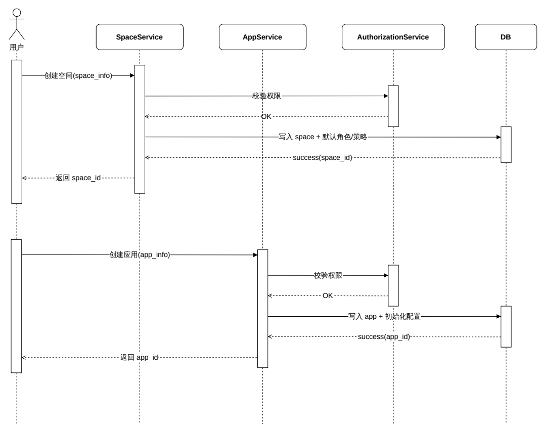
图 3-9: 空间与应用管理时序图
