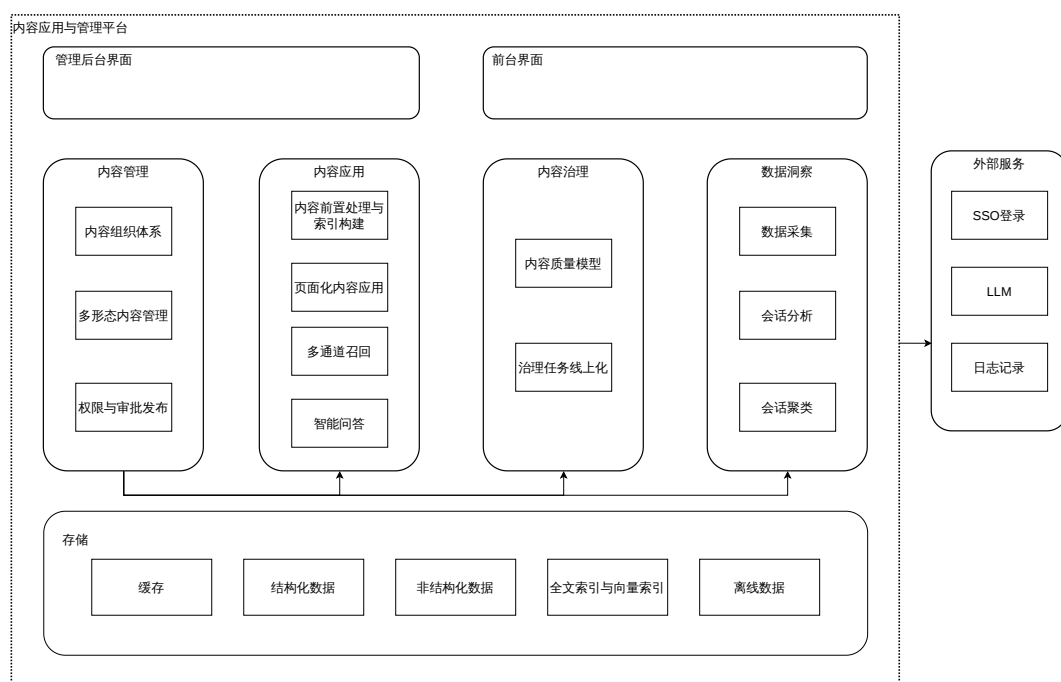
图 3-6: 逻辑视图
