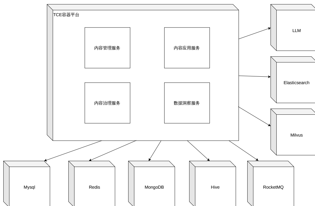
图 3-8: 物理视图
