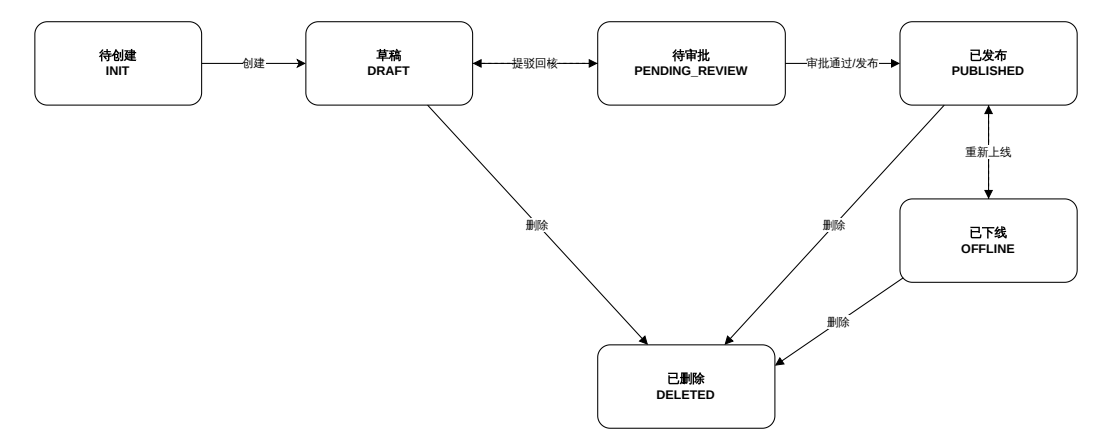
图 3-10: 内容状态机图
