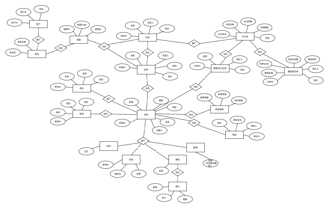
图 3-17: 数据库 E-R 图
