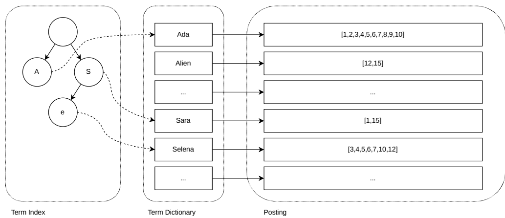
图 2-3: Elasticsearch 倒排索引示意图
