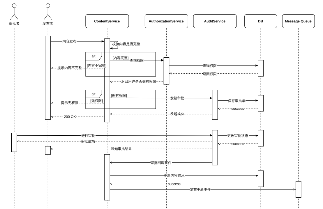
图 3-11: 内容发布流程时序图
