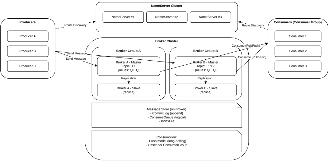
图 2-2: RocketMQ 架构图
