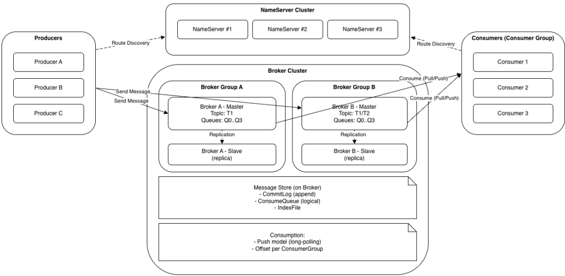
图 2-1: RocketMQ 架构图
