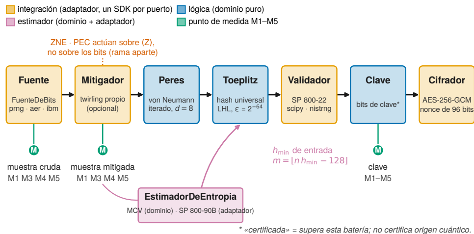
Figura 1. Pipeline: fuente de bits, mitigación, Peres, Toeplitz con LHL, validación y clave AES-256-GCM. Las métricas se miden en tres puntos (cruda, mitigada y clave). ZNE y PEC actúan sobre el valor esperado y no sobre los bits.
