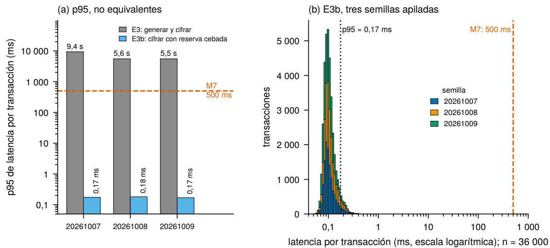
Figura 7. E3b: (a) percentil 95 de la latencia por transacción en E3 (generar y cifrar la clave) y en E3b (cifrar con una reserva ya cebada), escala logarítmica; las dos magnitudes no son equivalentes. (b) Distribución de las 36 000 latencias de E3b (tres semillas).
