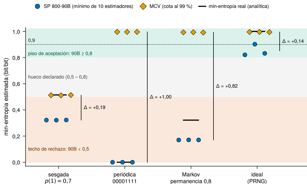
Figura 4. Control positivo: 90B frente a MCV para cada fuente sintética y semilla, con la entropía real analítica. Bandas: techo 0,5 (rechazo) y piso 0,8 (aceptación) del control P1.
