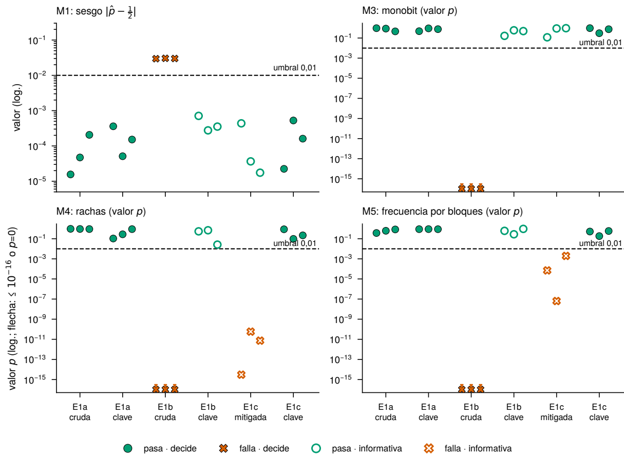
Figura 3. E1: M1, M3, M4 y M5 por semilla y punto de medida (C.E1a a C.E1c). Símbolo lleno: decide; hueco: informativo. Verde: pasa; bermellón: no pasa.
