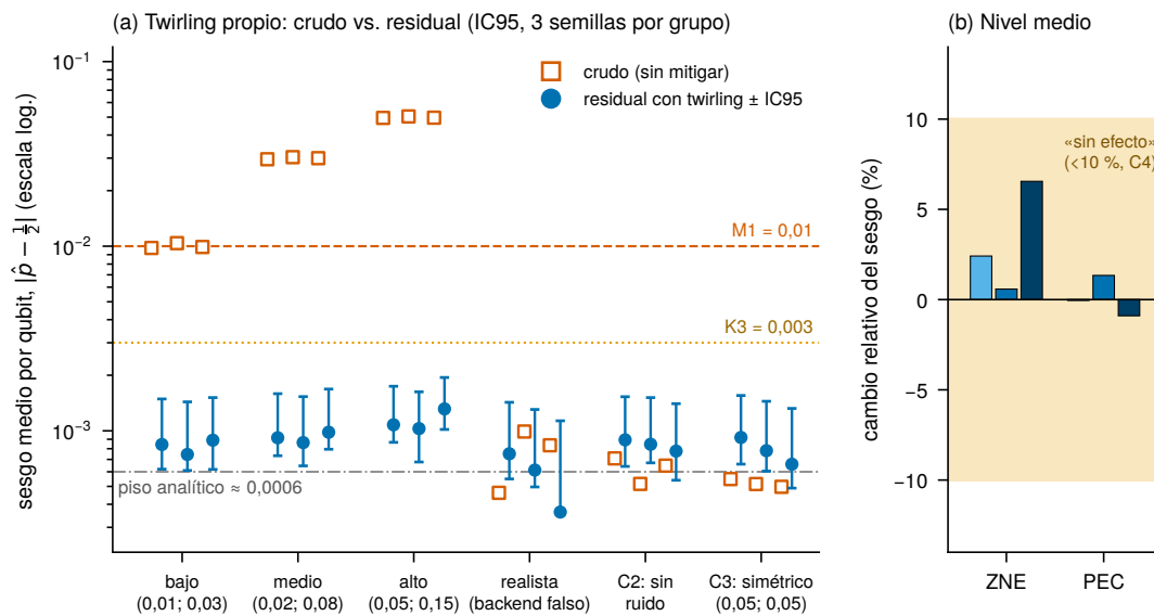
Figura 5. E2: (a) sesgo medio por qubit, crudo frente a residuo tras el twirling , por nivel de ruido y semilla, con IC95 y el umbral M1 (escala logarítmica); (b) cambio relativo del sesgo con ZNE y PEC en el nivel medio.
