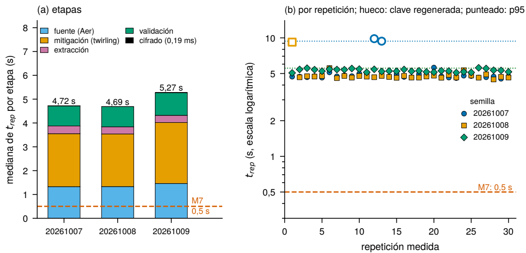
Figura 6. E3: (a) mediana del tiempo por etapa del ciclo completo, apilada, frente al umbral de M7; (b) t_{rep} de cada repetición medida (escala logarítmica), con el p95 de cada semilla (punteado) y las repeticiones con clave regenerada (hueco).
