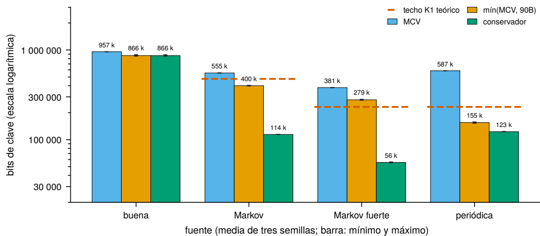
Figura 8. E5: bits de clave por fuente y dimensionado (media de tres semillas y rango), escala logarítmica. La marca horizontal es el techo teórico de cada fuente defectuosa.
