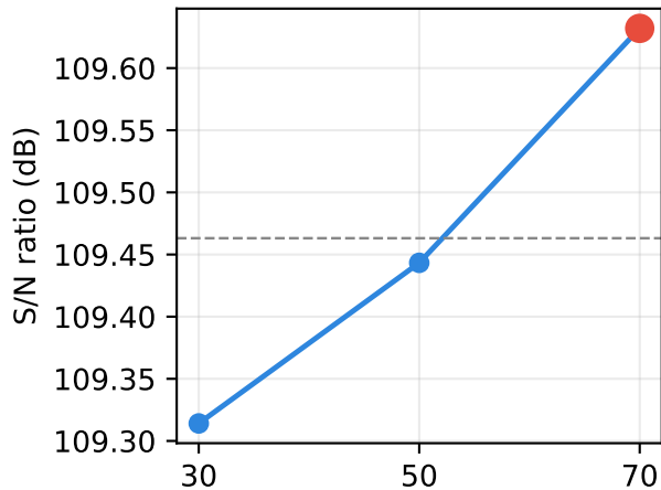
A: population N
