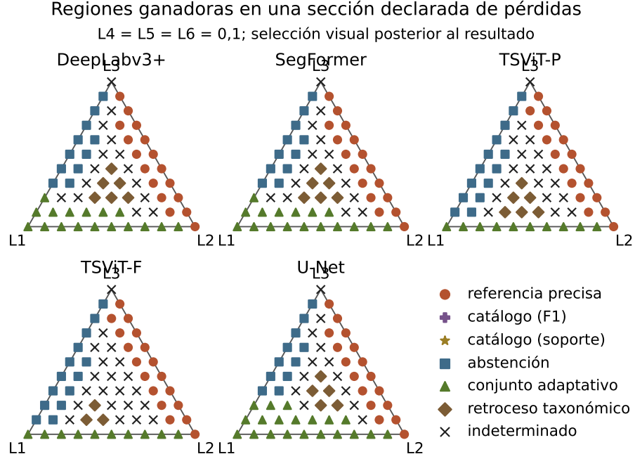
Figura 1. Regiones de ganador cierto en una sección declarada del atlas exploratorio PASTIS-R. Los símbolos identifican la acción ganadora; las cruces son evaluaciones donde la banda simultánea no establece una. Cada panel es un predictor congelado. Las acciones de restricción del catálogo permanecen en la leyenda aunque ninguna gane en esta sección, cerrando la cuenta de seis acciones. La sección mostrada es la primera de la enumeración congelada y fue elegida para presentación después de obtener resultados.
