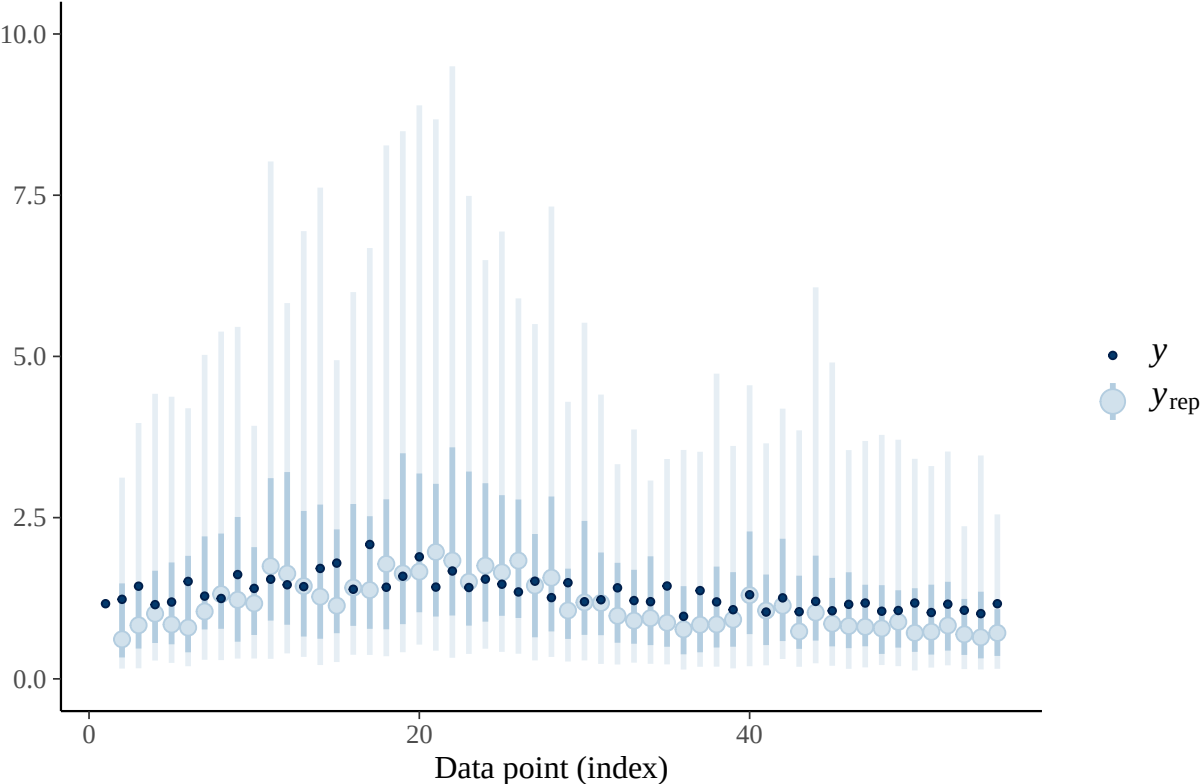
PPC: random walk q – CPUE timeseries
