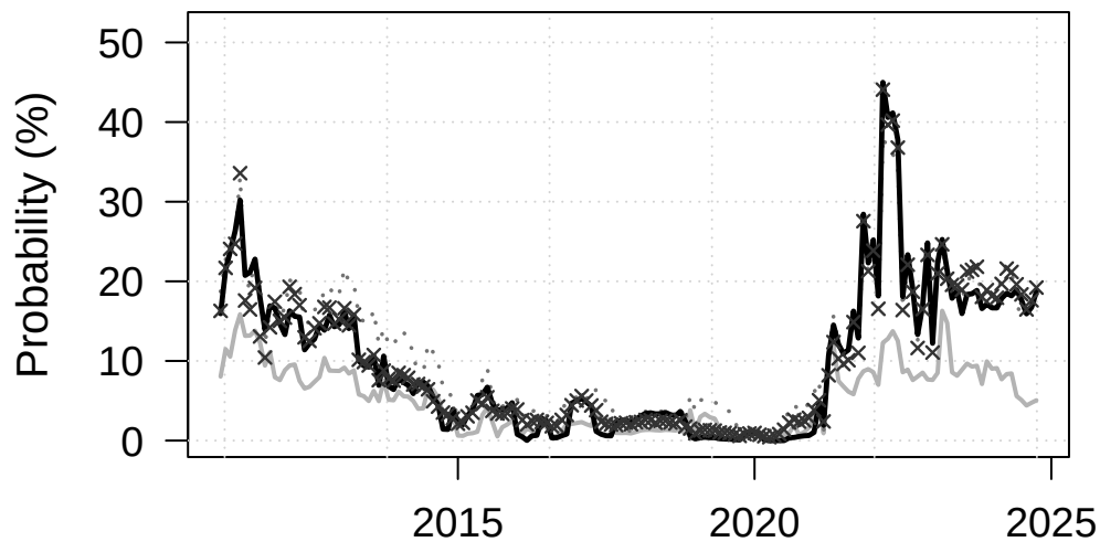
U.S., 5y
