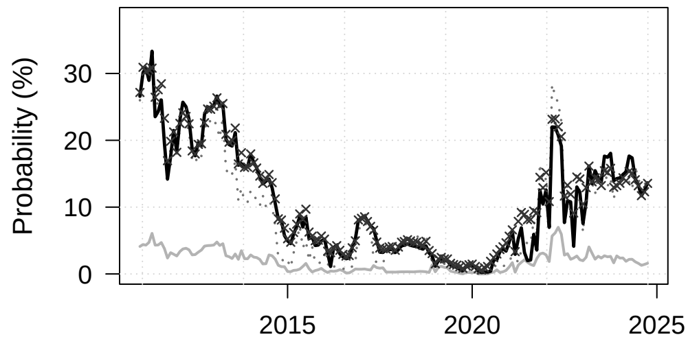
U.S., 10y
