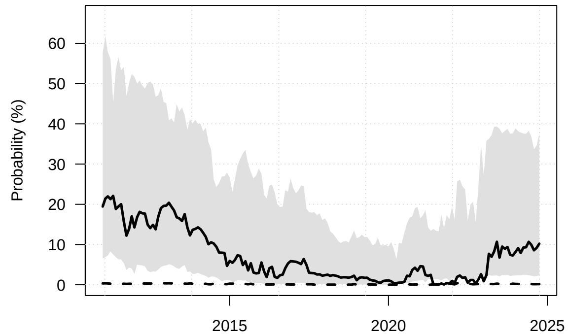
U.S., \pi > 5\%
