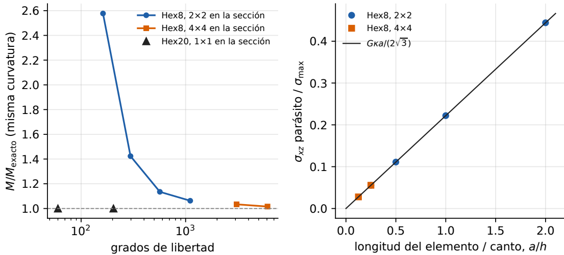
Figura 6.1: Izquierda: momento necesario para la misma curvatura, relativo al exacto, frente al número de grados de libertad. Derecha: esfuerzo cortante parásito en los puntos de Gauss del Hex8 frente a la longitud del elemento; la recta es la fórmula del texto.
