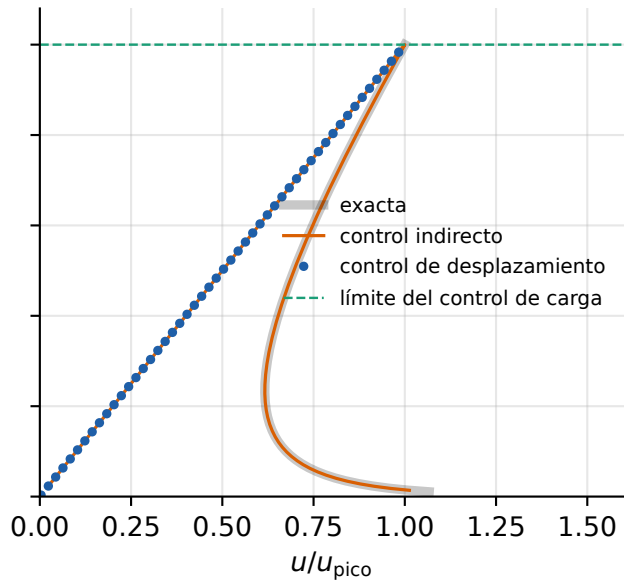
barra larga ( L = 1 m, 10 elementos)
